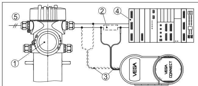
Figura 22: Collegamento del PC via HART alla linea del segnale
