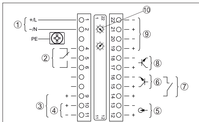
Figura 10: Vano dell'elettronica e di connessione negli apparecchi non-Ex e negli apparecchi con uscita in corrente senza sicurezza intrinseca
