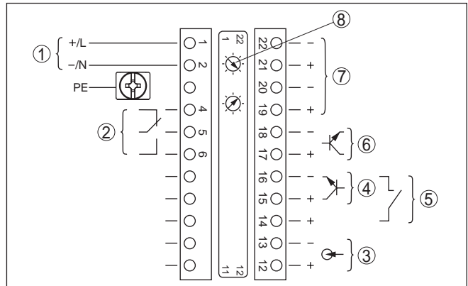
Figura 12: Vano dell'elettronica e di connessione (Ex-d) per apparecchi con uscita in corrente a sicurezza intrinseca
