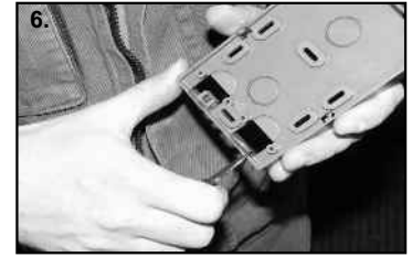
6. Eseguire nella parte posteriore un passaggio per il cavo di collegamento.
