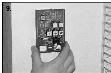
9. Montare l'elettronica del comando sugli arresti del coperchio.
