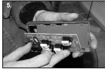
5. Togliere l'elettronica dalla parte posteriore del comando.
