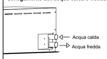
Collegamento dell'acqua calda e fredda
