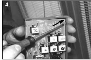
4. Con un cacciavite spingere attentamente sugli arresti nei fianchi del comando.
