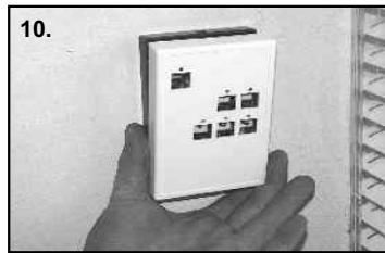
10. Montare la parte anteriore del pannello di comando sugli arresti inferiori della parte posteriore del pannello e "fare clic".
