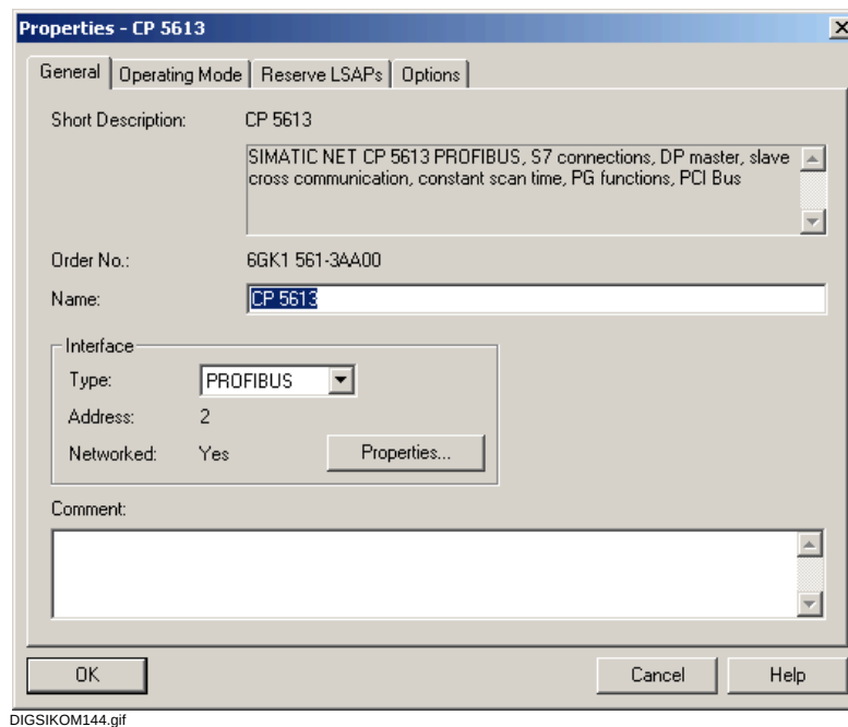
Fig. 7-46 Proprietà - CP 5613
