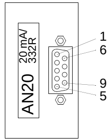
Fig. 2-33 connettore DSUB a 9 poli
