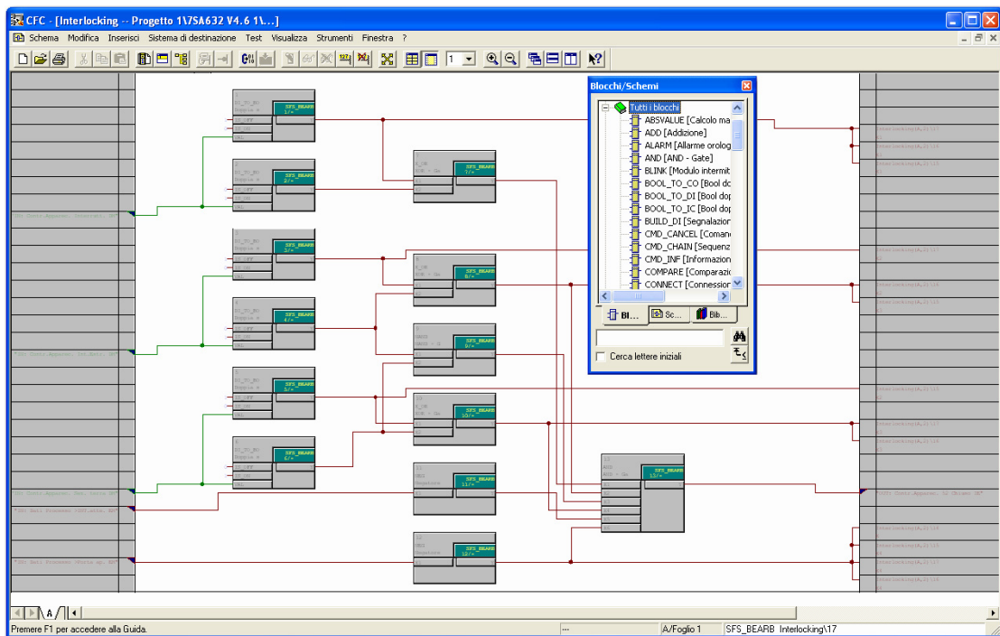
Fig. 5-34 DIGSI 4 CFC
