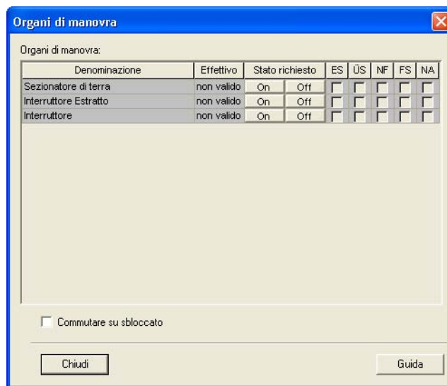
Fig. 6-55 Comando DIGSI 4
