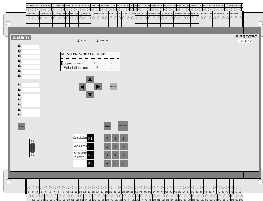
Fig. 2-11 Display a 4 righe, Dimensioni custodia 1_{I1} , esempio di montaggio sporgente senza collegamenti per conduttori a fibre ottiche
