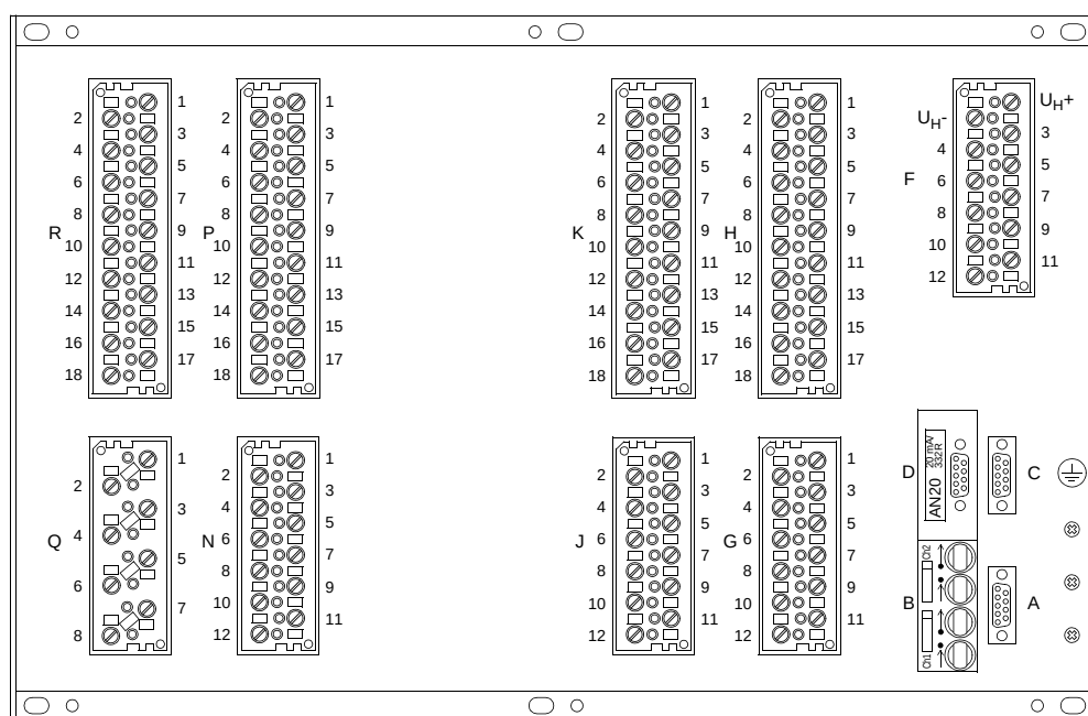
Fig. 2-6 Esempio di vista posteriore, dimensioni custodia 1/1
