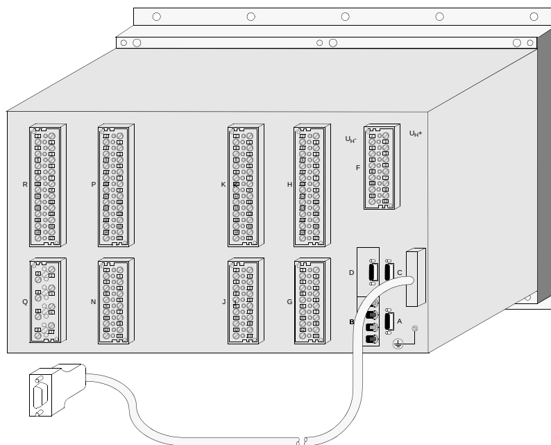
Fig. 2-17 Dispositivo SIPROTEC 4 , dimensioni custodia \frac{1}{1} con cavo Dongle, esempio
