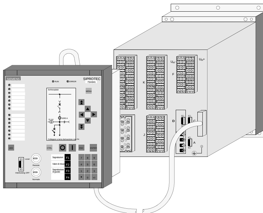
Fig. 2-14 Dispositivo SIPROTEC 4 con unità di comando separata, dimensioni custodia 1\frac{1}{2} , esempio
