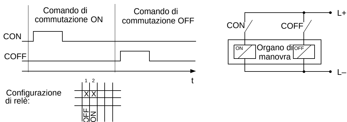
Fig. B-5 Comando doppio unipolare
