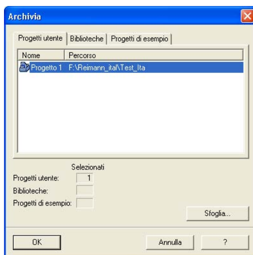
Fig. 4-15 Archiviazione
