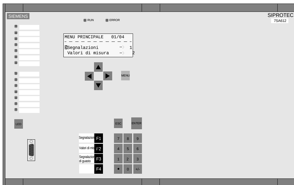
Fig. 2-5 Display a 4 righe, Dimensioni custodia 1/1 , esempio di montaggio incassato e in armadio
