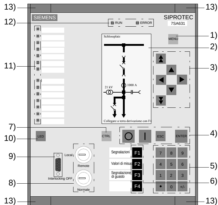
Fig. 2-2 Esempio di vista frontale, dimensioni custodia 1\frac{1}{2}
