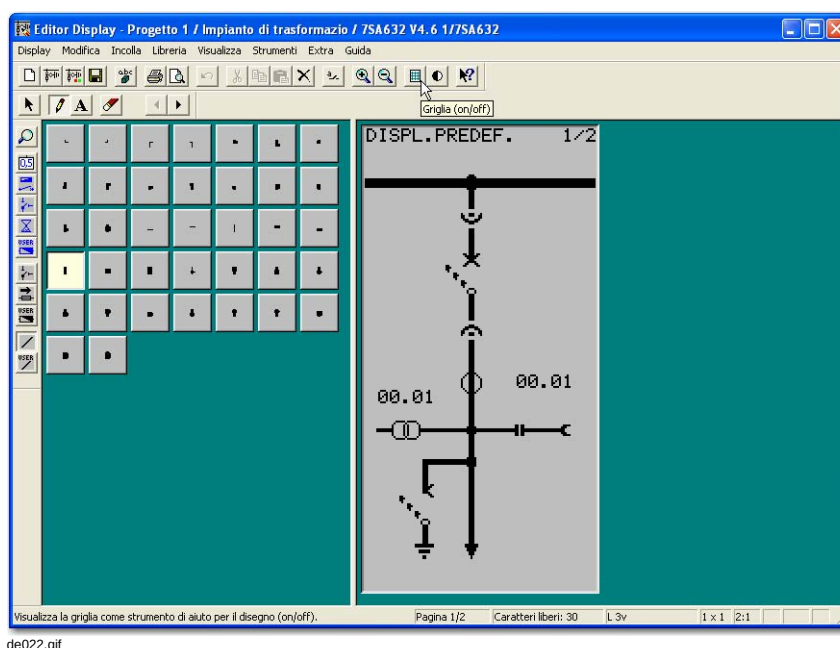
Fig. 5-58 Griglia nascosta
