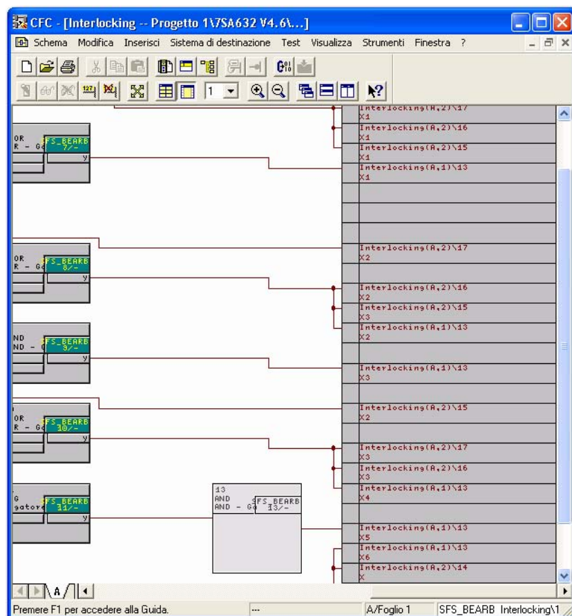
Fig. 5-12 Esempio di configurazione CFC, connessioni delle grandezze di uscita
