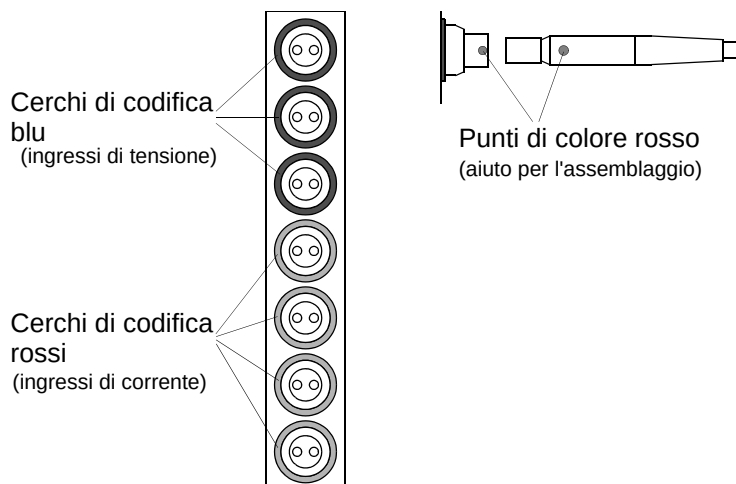
Fig. 2-35 Prese del dispositivo
