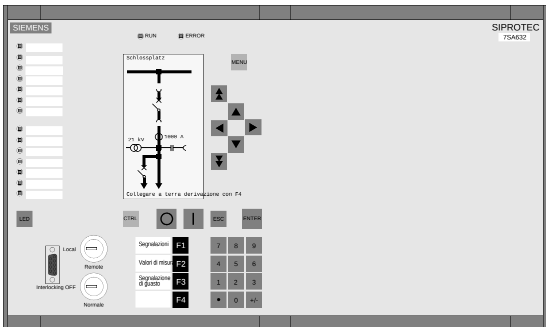
Fig. 2-8 Display grafico, Dimensioni custodia 1/1 , esempio di montaggio incassato e in armadio
