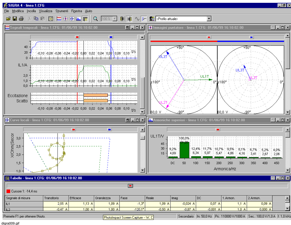
Fig. 6-30 Esempio di valutazione delle registrazioni dei guasti su SIGRA 4
