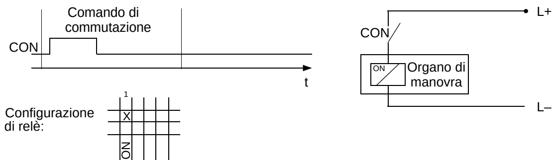
Fig. B-4 Comando semplice unipolare
