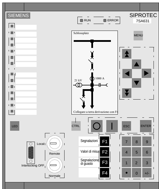
Fig. 2-7 Display grafico, Dimensioni custodia 1/2 , esempio di montaggio incassato e in armadio
