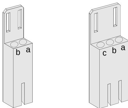
Fig. 2-26 Connettore bipolare e tripolare
