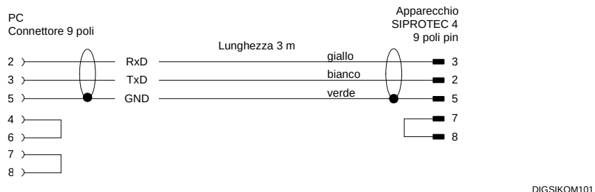
Fig. A-6 Schema di collegamento del cavo 7XV5100-4 tra computer e SIPROTEC 4
