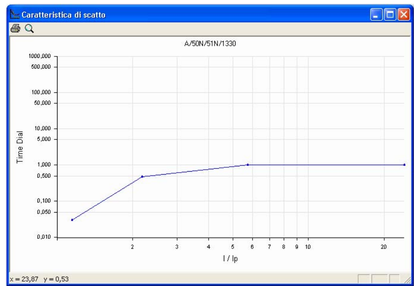
Fig. 5-85 Caratteristica
