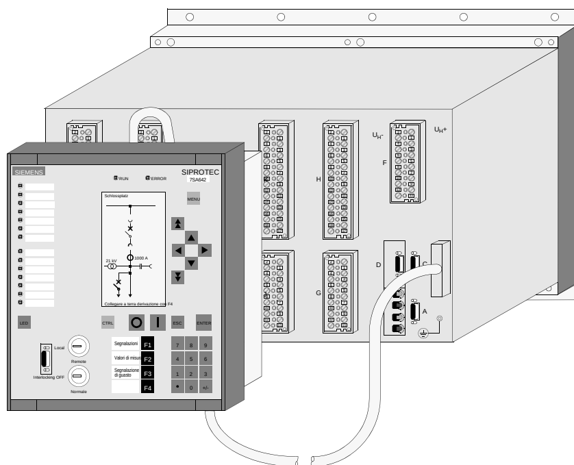
Fig. 2-15 Dispositivo SIPROTEC 4 con unità di comando separata, dimensioni custodia 1\frac{1}{1} , esempio
