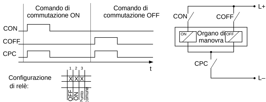
Fig. B-6 Comando doppio 1 \frac{1}{2} poli
