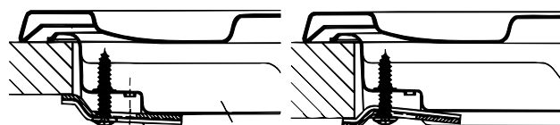
Position du crochet pour plan H=20mm
