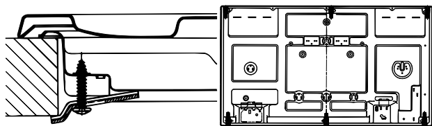
Posizione gancio per top H=40mm
