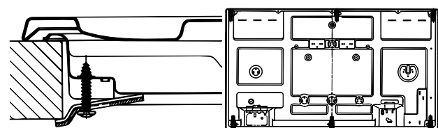
Position du crochet pour plan H=40mm
