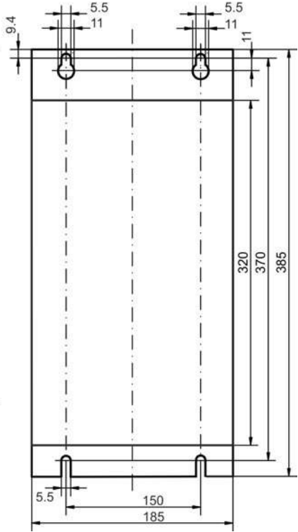
AKD larghezza estesa 480V, 48A
