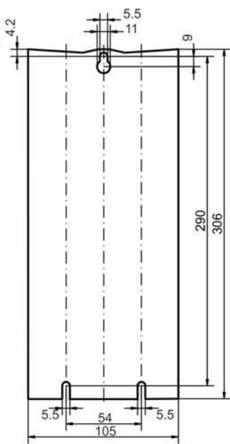
AKD larghezza estesa 480V, 24A
