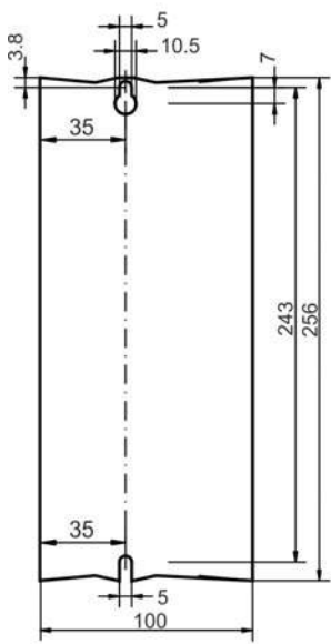
AKD larghezza estesa 480V, 3A - 12A
