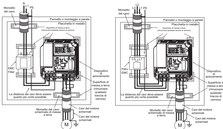
Cablaggio conforme agli standard EMC di unità monofase e trifase
