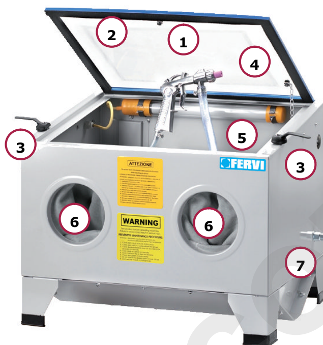
Figura 2 - Parti principali della sabbiatrice.
