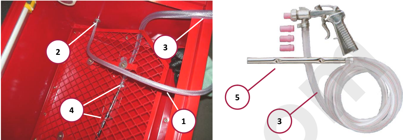
Figura 5 - Collegamento della pistola sabbiatrica.
