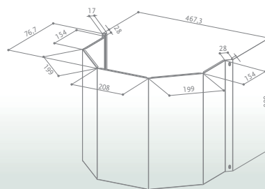
KIT PREMIO ANGOLO H990 X
