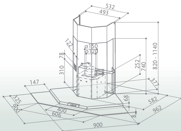
PREMIO ANGOLO/SP 90 cm
