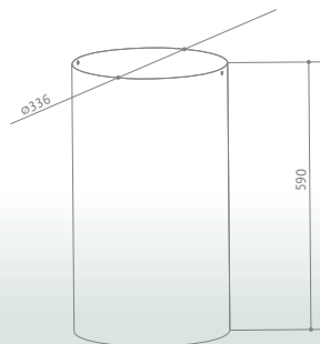
KIT ISOLA H590 D340 X
