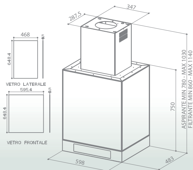
GLORY ISOLA - MAIN ISOLA
