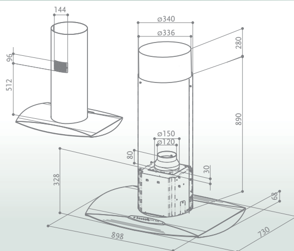
AXIA PLUS ISOLA
