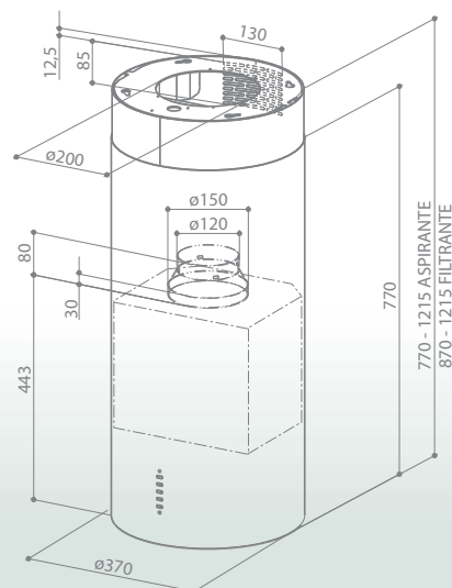
CYLINDRA ISOLA - CYLINDRA ISOLA GLOSS
