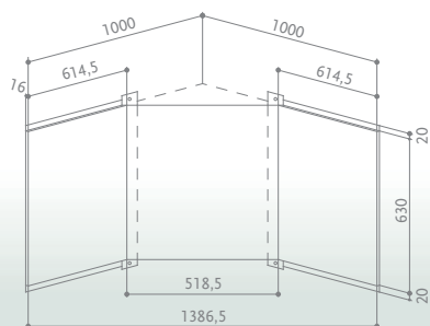
KIT FONDALE PREMIO ANGOLO X
