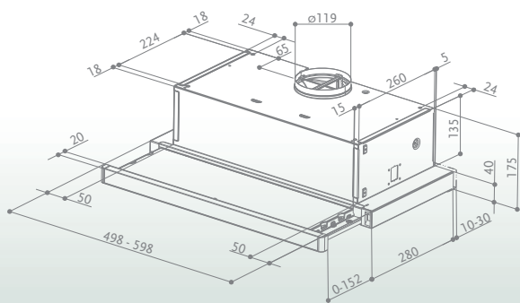
FLEXA - FLEXA VITRO
