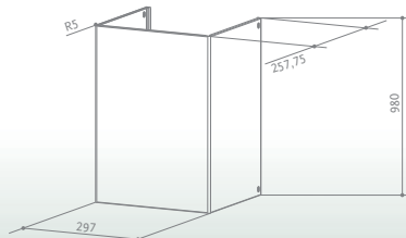
KIT ALTO H990 AL
