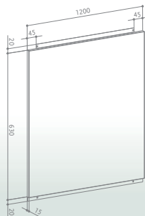
KIT FONDALE 120X63 P.15 X
