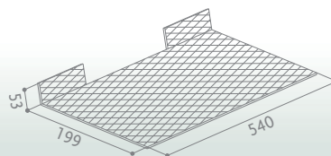
CONF.1 FILTRO ESTRAIBILI 60
