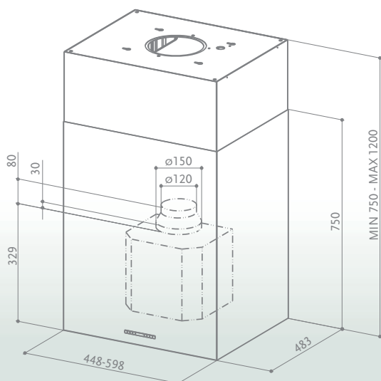
CUBIA ISOLA GLOSS
