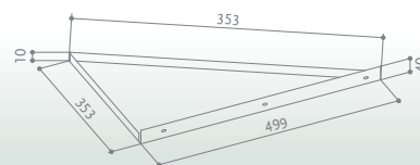
KIT ADATTATORE ANGOLO X
