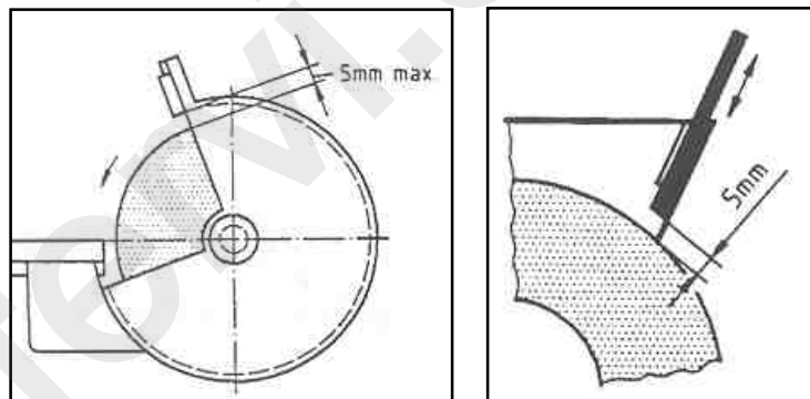
Figura 6 – Regolazione degli schermi di protezione.
