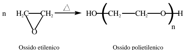
Figura 12. Polimerizzazione dell'ossido etilenico in ossido polietilenico
