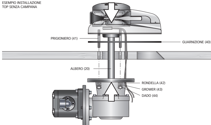
ESEMPIO INSTALLAZIONE TOP SENZA CAMPANA
