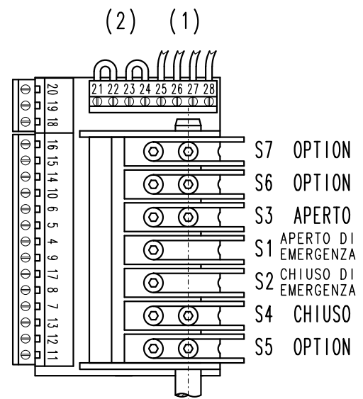
Fig. 2: Contattiera di fine corsa
