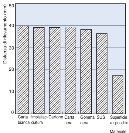
E3Z-LL□3/-LL□8
