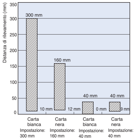
E3Z-LL□1/-LL□6
