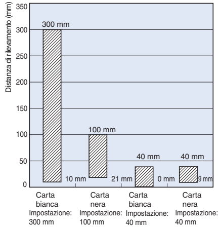
E3Z-LL□3/-LL□8
