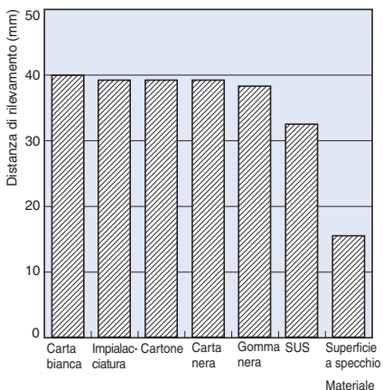
E3Z-LL□1/-LL□6
