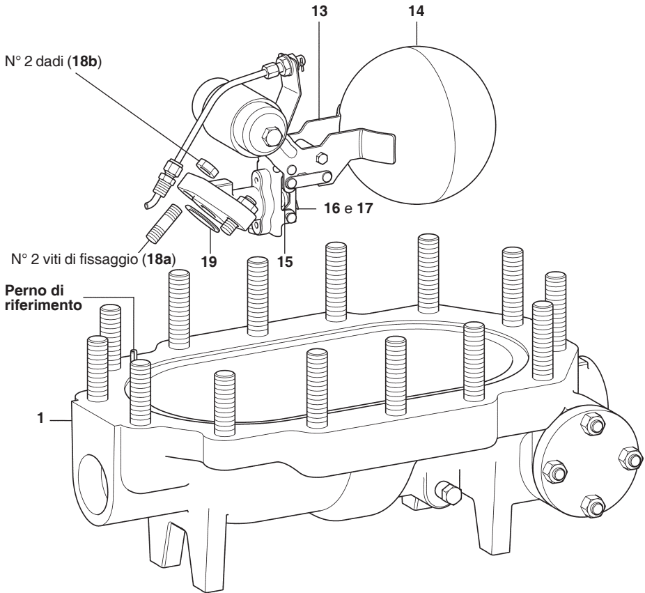
Fig. 7 - Smontaggio del gruppo meccanico di scarico
