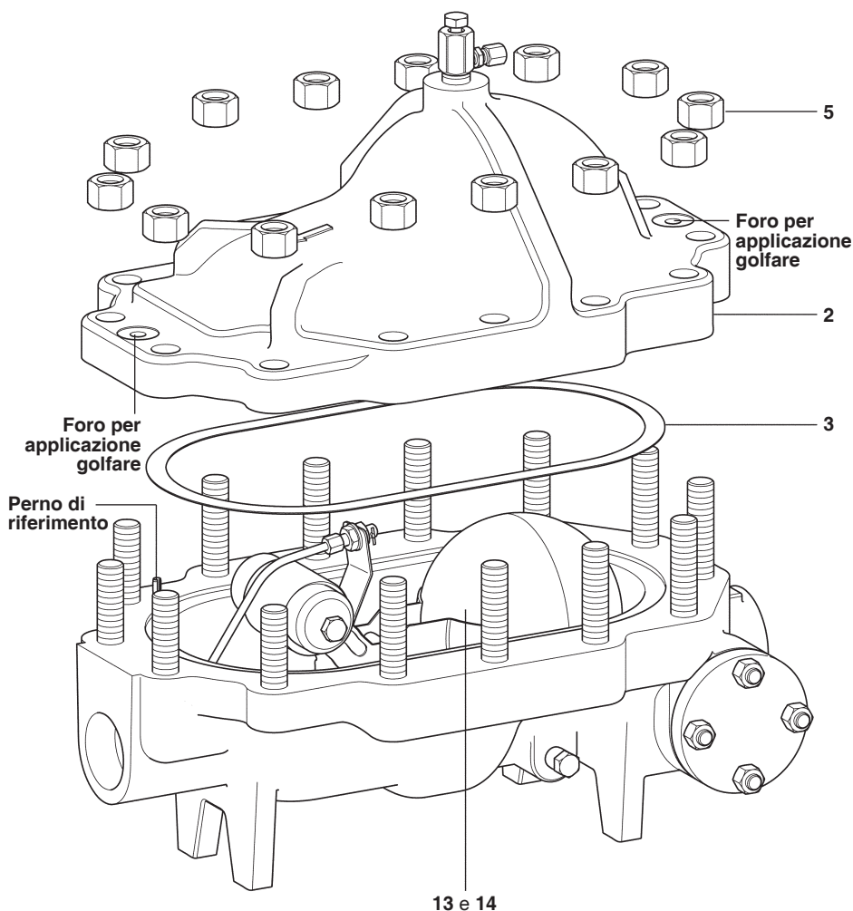
Fig. 6 - Smontaggio del coperchio
