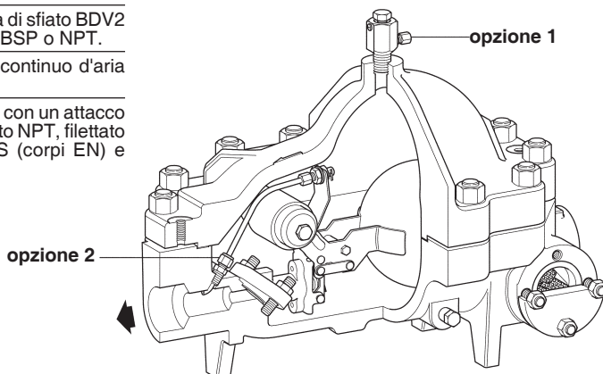
Fig. 1 - Scaricatore FTC80 (R-L) da 1 1/2" e 2" con attacchi a tasca a saldare
