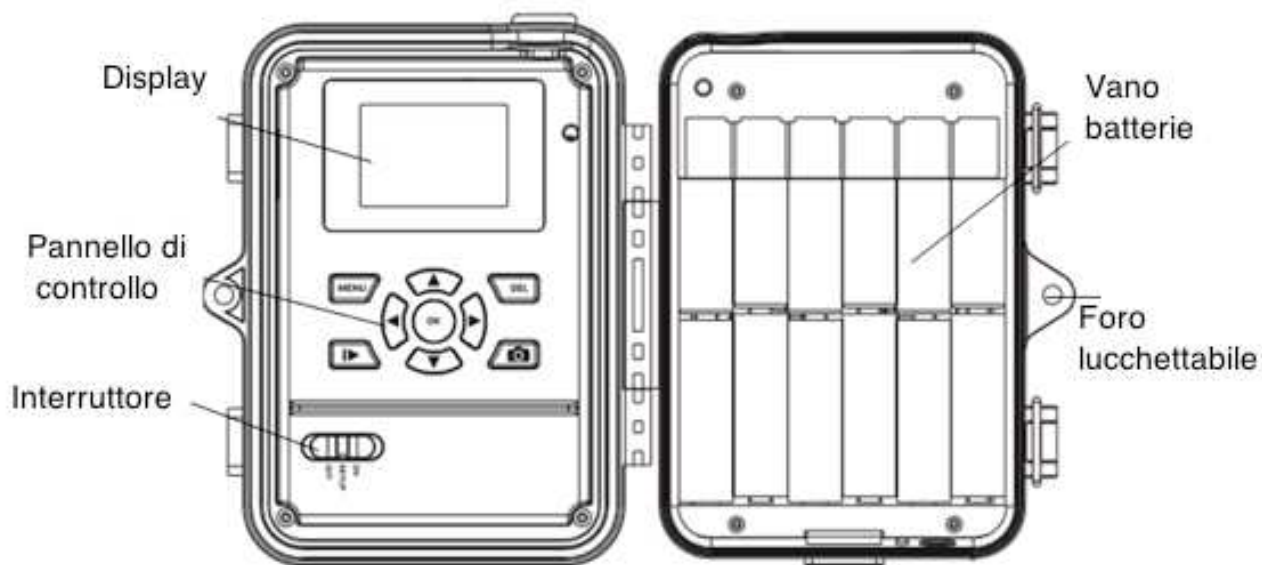
Fig 2: Interfaccia operativa
