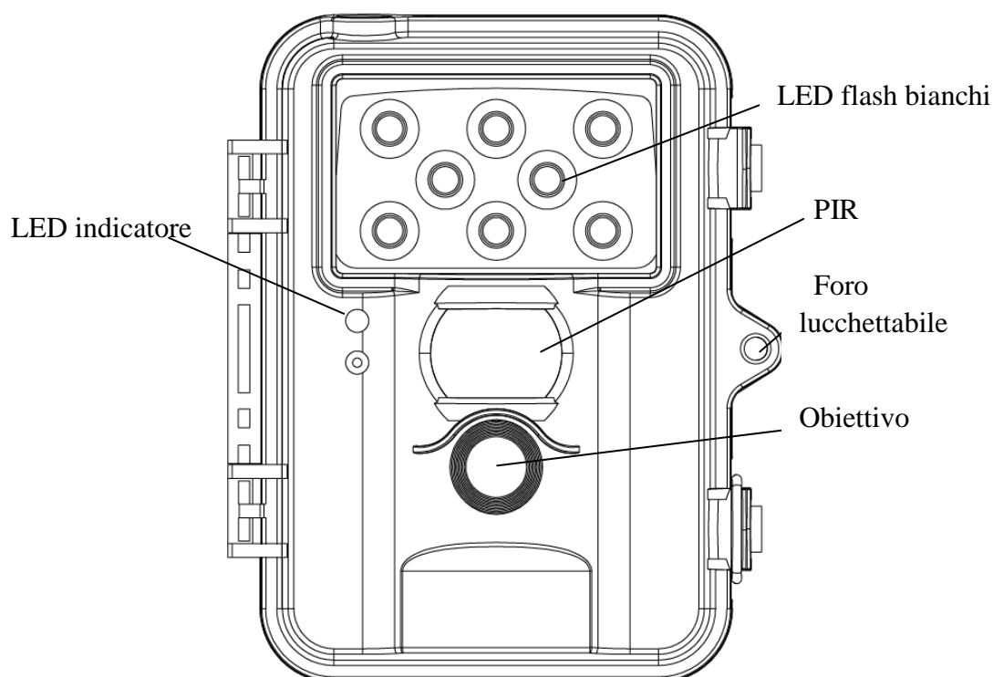
Fig 1: Vista frontale
