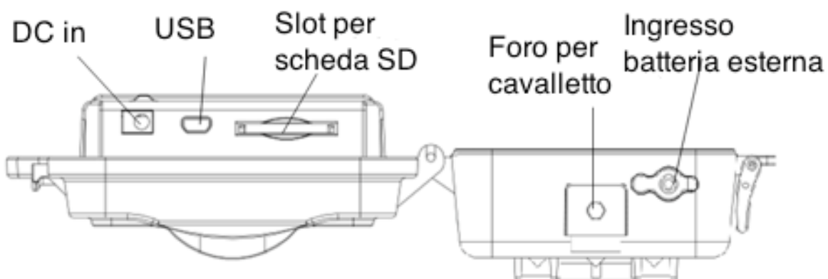
Fig 3: Vista inferiore
