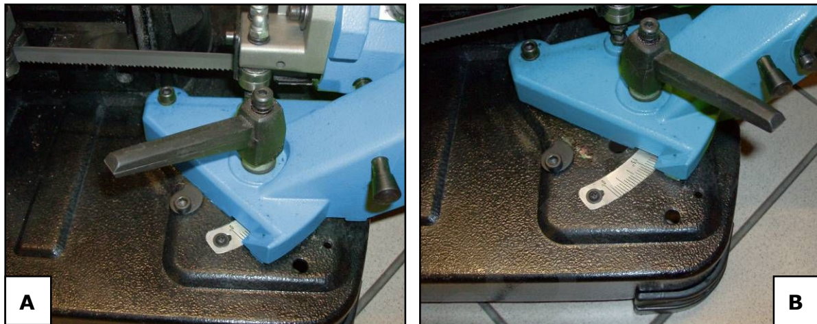
Figura 5 – Leva di bloccaggio della testa.
