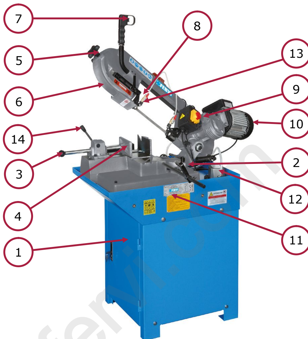
Figura 1 – Dettaglio delle parti principali della segatrice.
