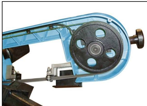
Figura 23 – Dettaglio lama.
