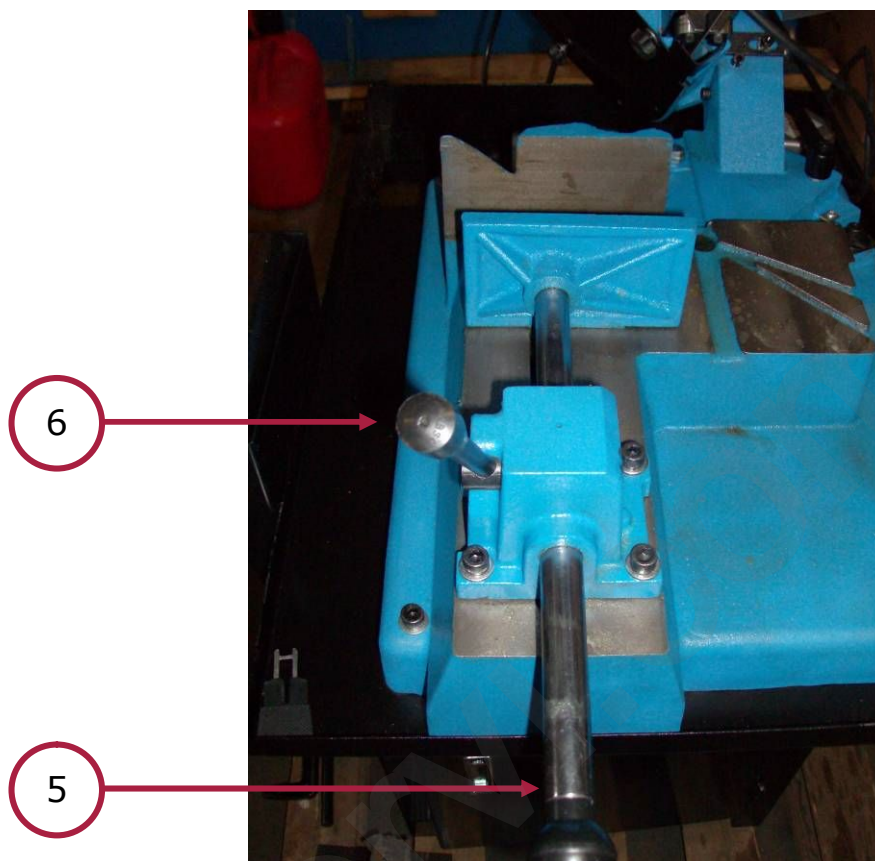
Figura 7 – Morsa di bloccaggio del pezzo.
