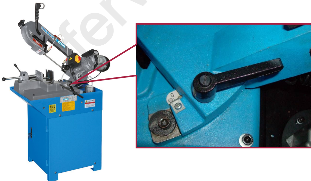
Figura 18 – Regolazione della posizione della testa.
