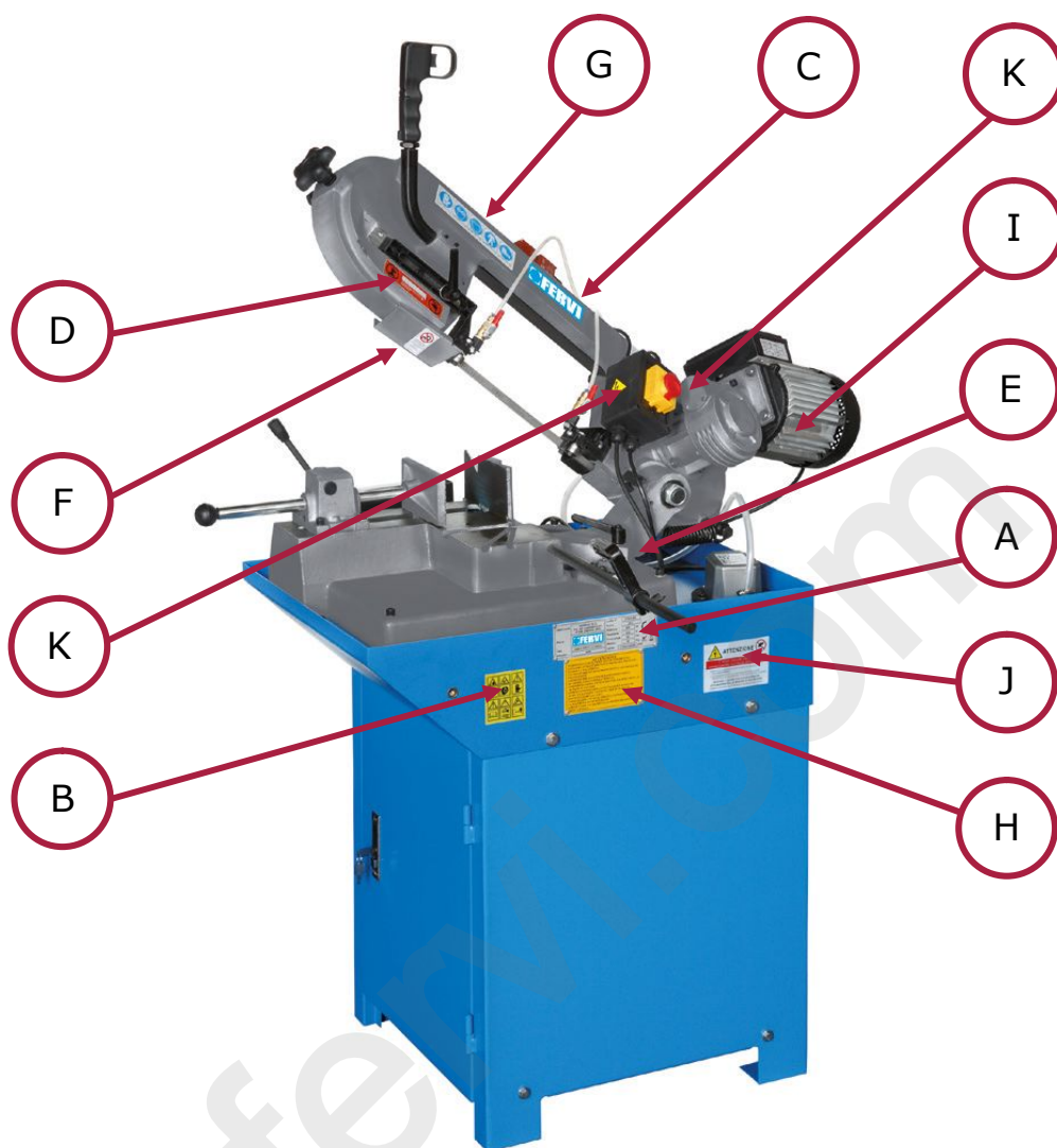
Figura 2 – Posizione delle targhe e dei pittogrammi.
