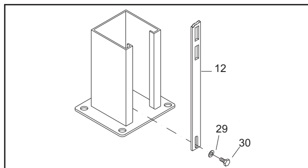
Fig.51 Bloccaggio dell'asta di sicurezza Fig.51 Safety rod locking
