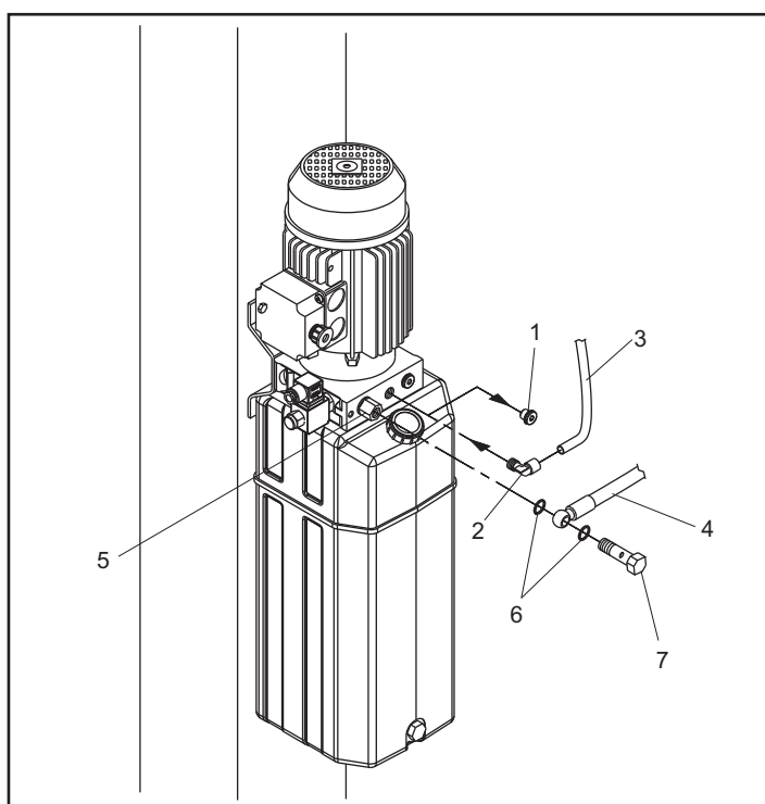
Fig.53 Allacciamento impianto idraulico
