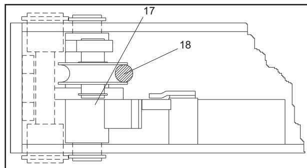
Fig.52 Posizionamento dei sensori fune Fig.52 Positioning of lifting cable sensors
