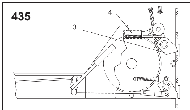
Fig.29 Martelletto di sicurezza e finecorsa mod.435 Fig.29 Safety wedge and limit switch model 435
