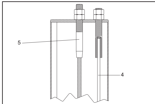
Fig.5 Sommità colonne Fig.5 Post top
