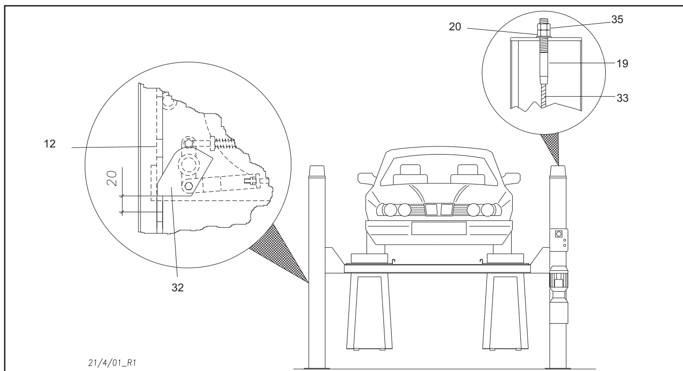
Fig.64 Registrazione funi
