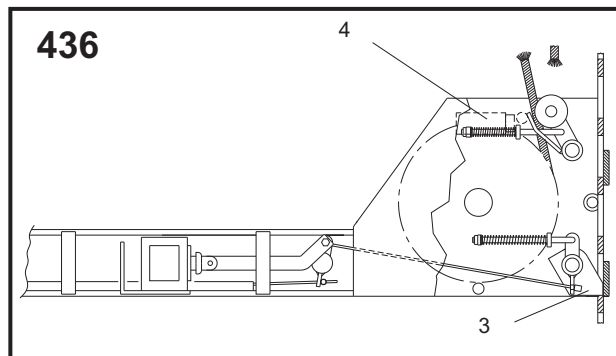
Fig.30 Martelletto di sicurezza e finecorsa mod.436 Fig.30 Safety wedge and limit switch model 436
