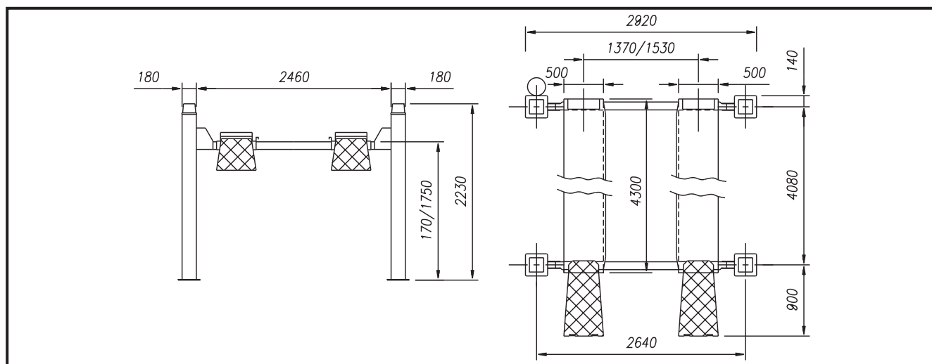
Fig.13 Dimensioni ed ingombri
