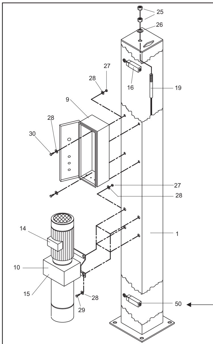
Fig.49 Preparazione colonna 1
