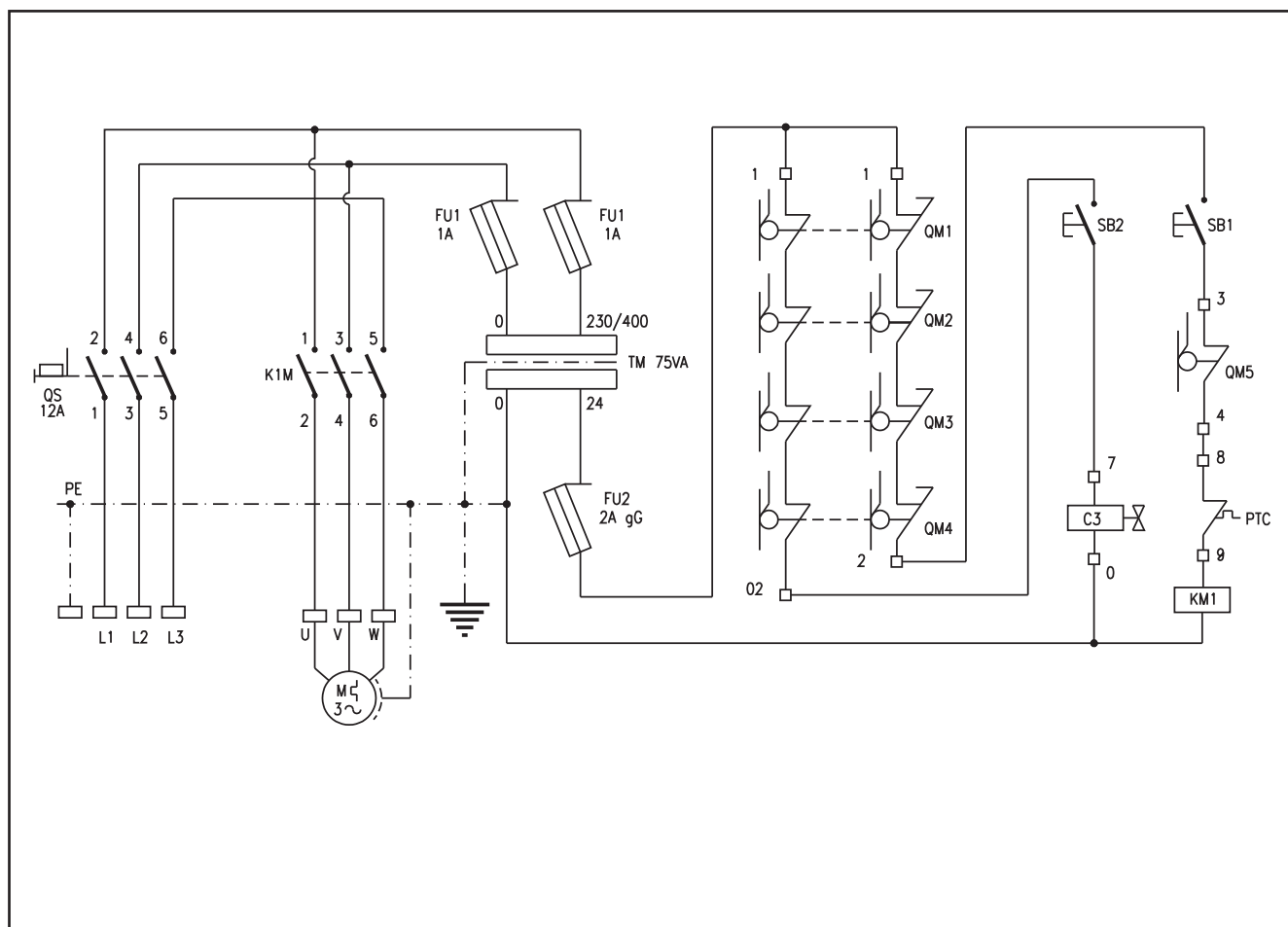
Schema elettrico 435
