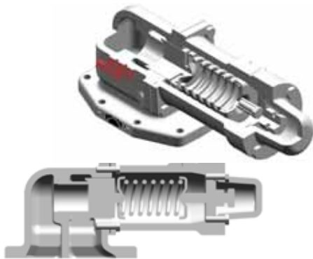
Valvola di by-pass – orizzontale
