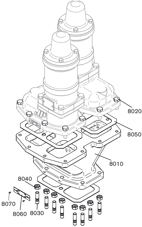
Doppia valvola di by-pass – verticale
