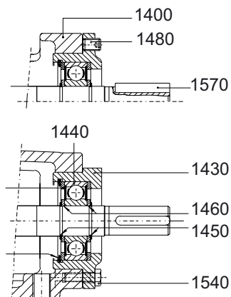
Smontaggio e montaggio del cuscinetto delle pompe TGGS 2-25/3-32/6-40
