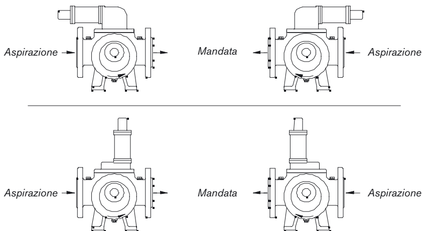
Installazione della valvola di by-pass
