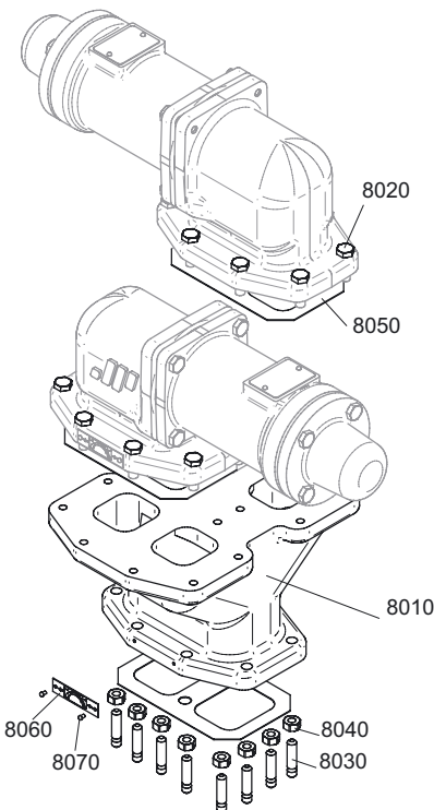
Doppia valvola di by-pass – orizzontale
