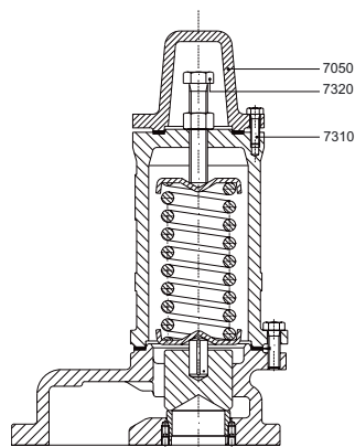
Valvola di by-pass verticale
