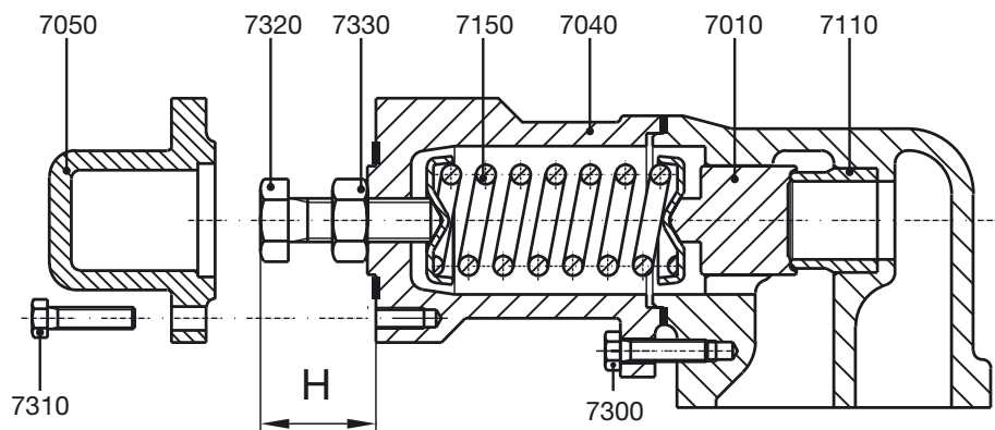
Montaggio e smontaggio della valvola di sicurezza
