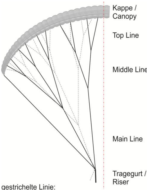
Fig 1 : CAD disegno del Mistral 7
