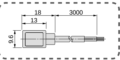
Dimensioni comuni
