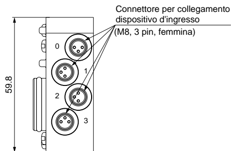
Assegnazione dei pin del connettore per la connessione del dispositivo d'ingresso (M8, 3 pin, femmina)
