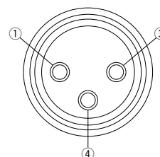
Assegnazione dei pin del connettore per la connessione del dispositivo d'ingresso (M8, 3 pin, femmina)
