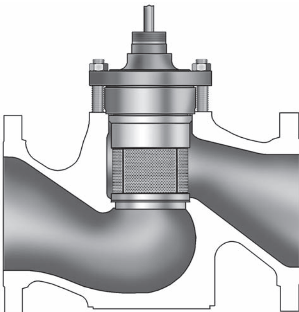
Figura 2. Sezione in dettaglio del trim WhisperFlo Fisher, corpo valvola tipico
