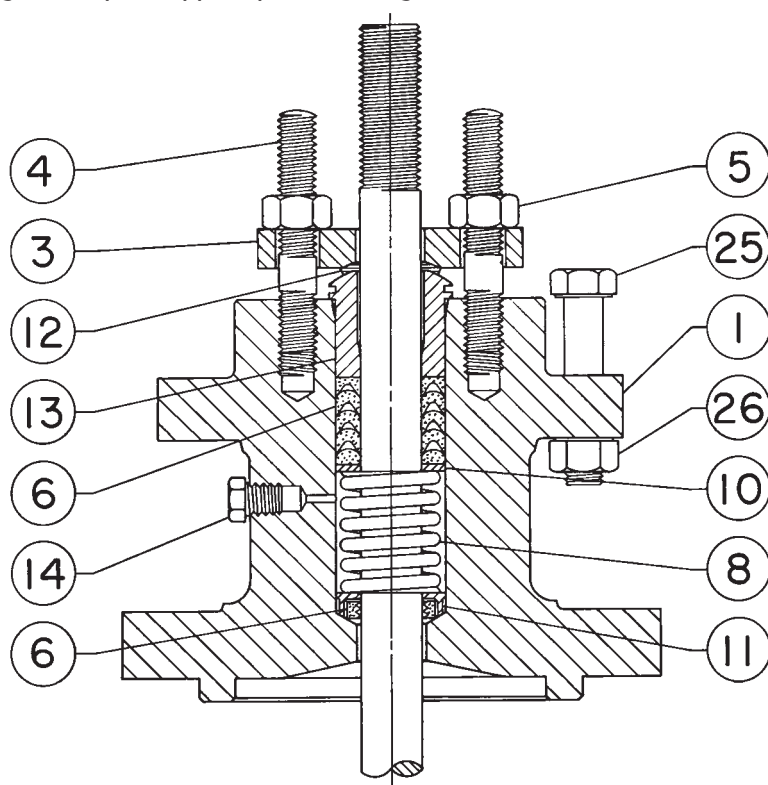
Figura 5. Tipico cappello per valvola a globo
