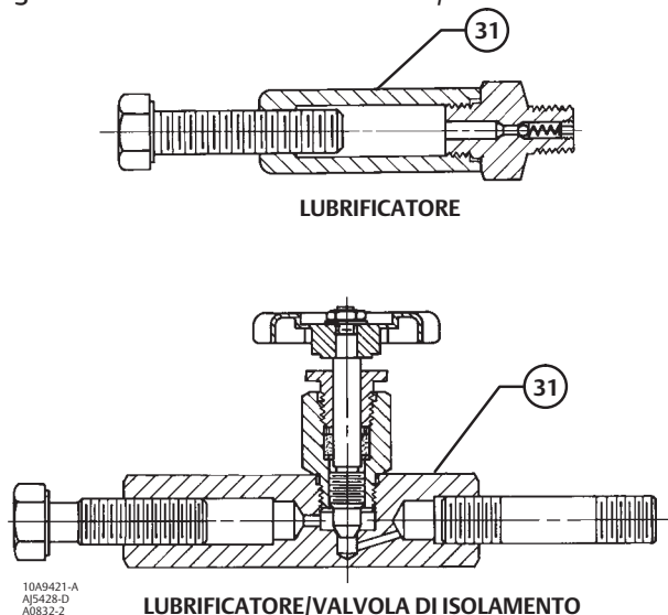
Figura 3. Lubrificatore e lubrificatore/valvola di isolamento
