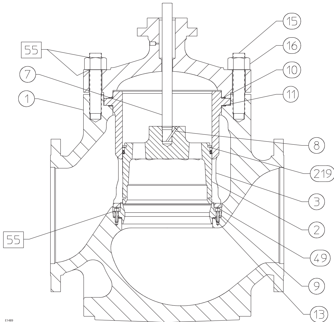
Figura 9. Tipica valvola EUT o EWT Fisher con opzione HTS1
