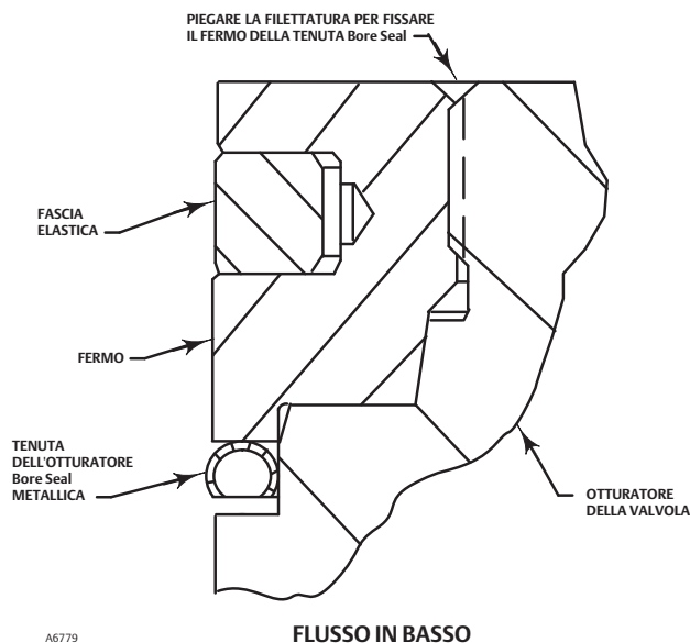
Figura 12. Piegatura delle filettature del fermo della tenuta Bore Seal
