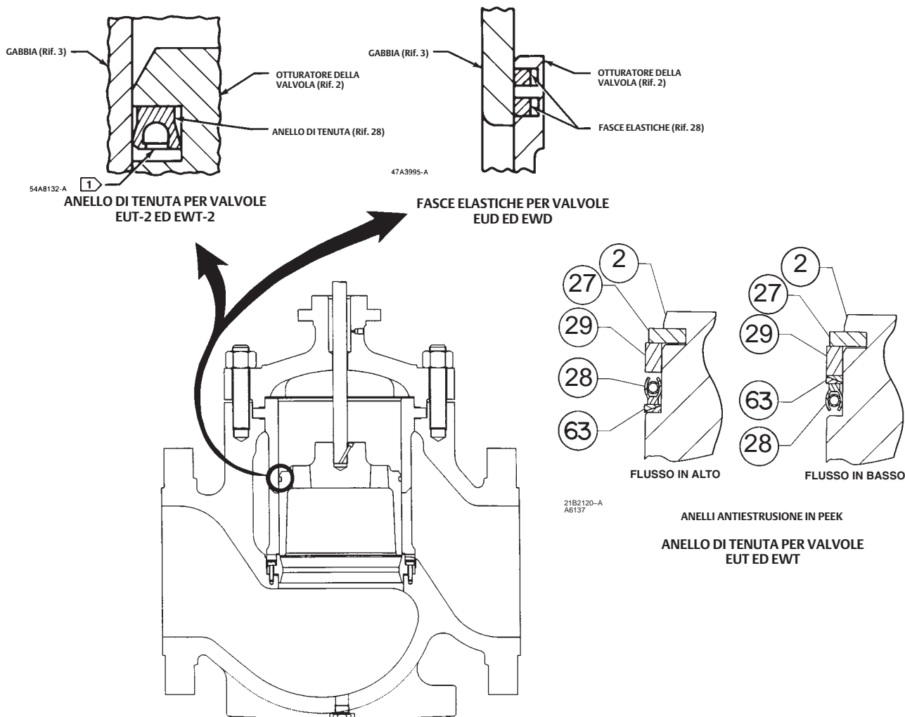
Figura 6. Dettagli dell'anello di tenuta e della fascia elastica
