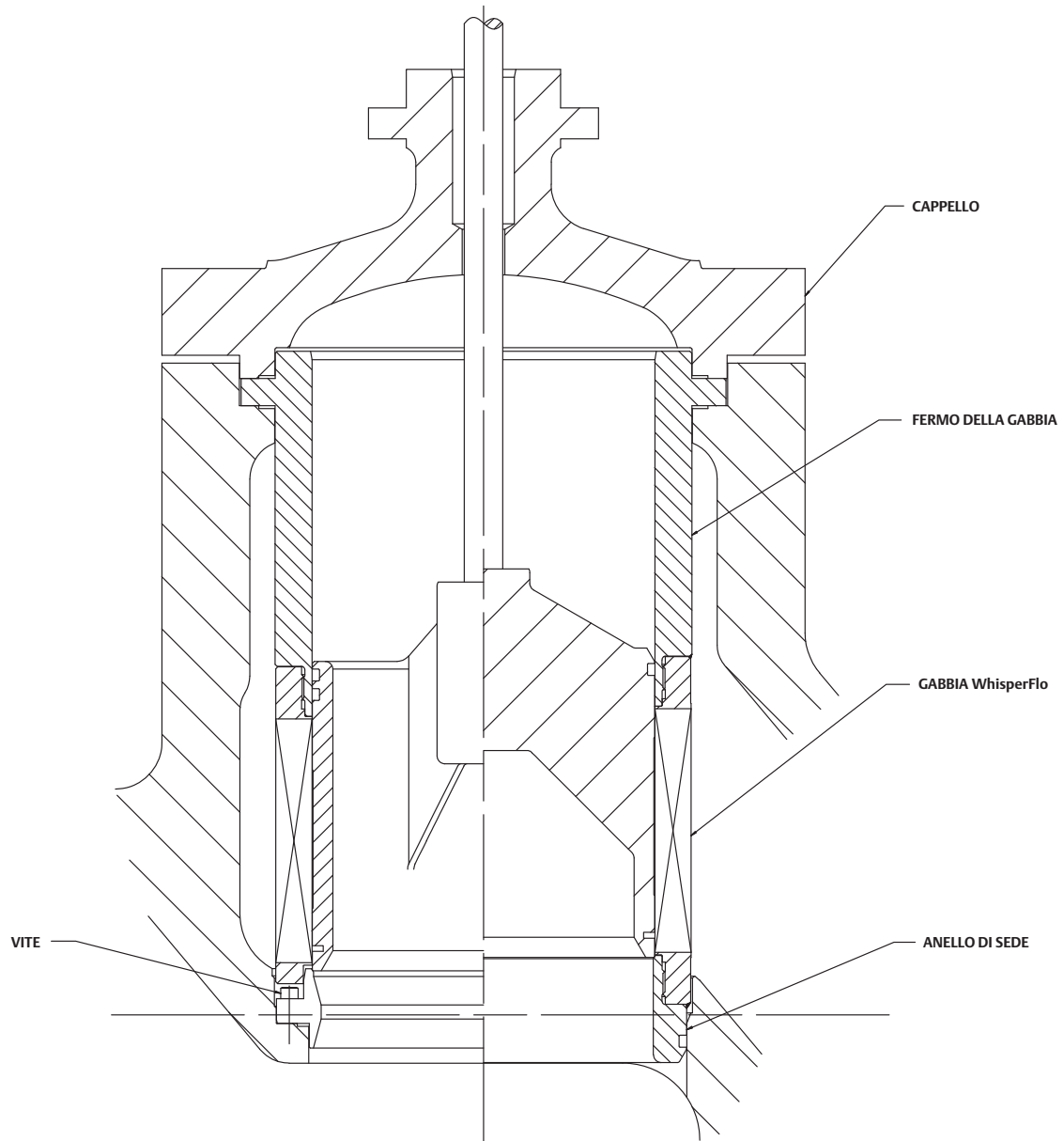
Figura 14. Tipici trim WhisperFlo Fisher
