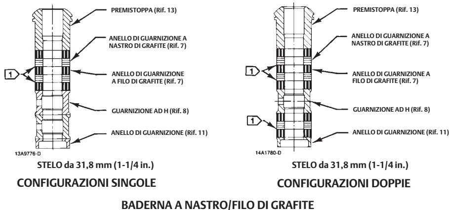
Figura 4. Baderna tipica (continua)
