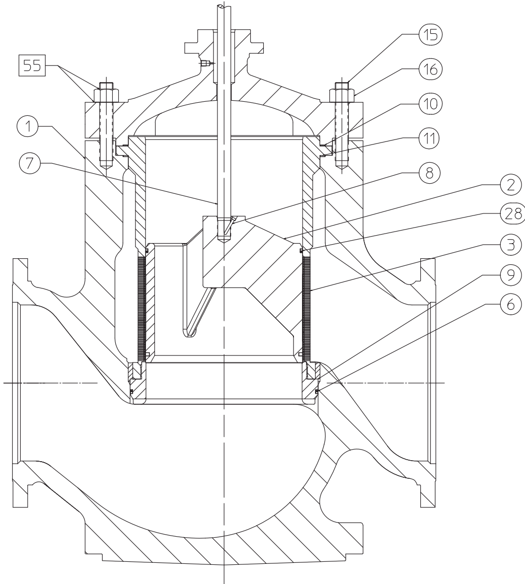
Figura 7. Tipica valvola EUT-2 o EWT-2 Fisher
