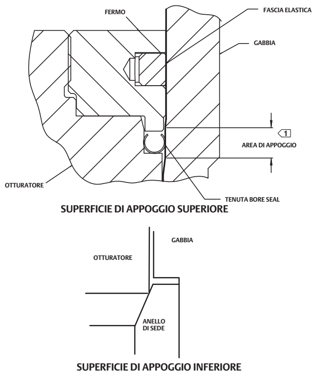
Figura 13. Superfici di appoggio inferiore (otturatore della valvola-anello di sede) e superiore (tenuta Bore Seal-gabbia)
