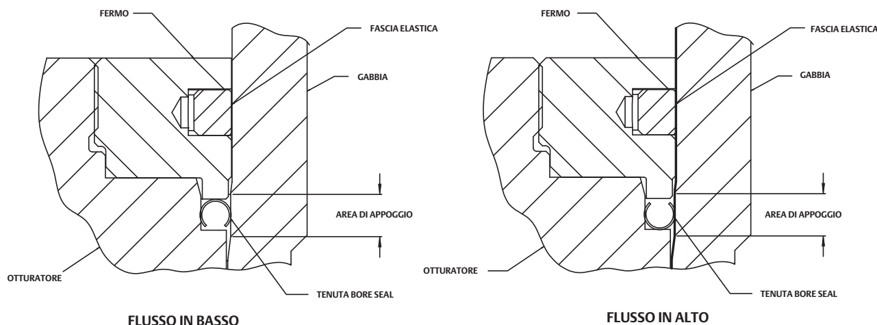
Figura 10. Valvola EUD ed EWD Fisher con trim Bore Seal
