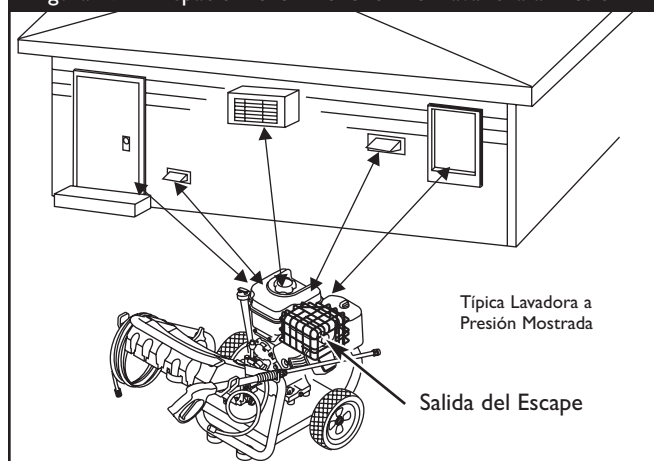
Figura 17 — Espacio Libre Alrededor del Lavadora a Presión
