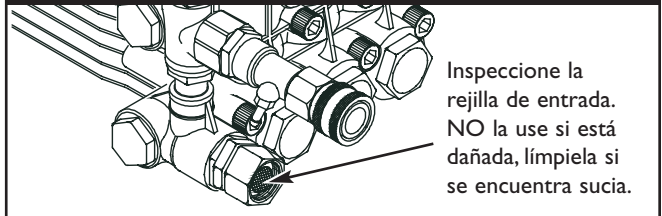
Figura 16 - Conecte la Manguera para el Jardín, a la Entrada de Agua
