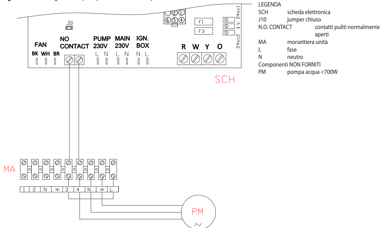
Figura 4.6 – Collegamento pompa circolazione acqua
