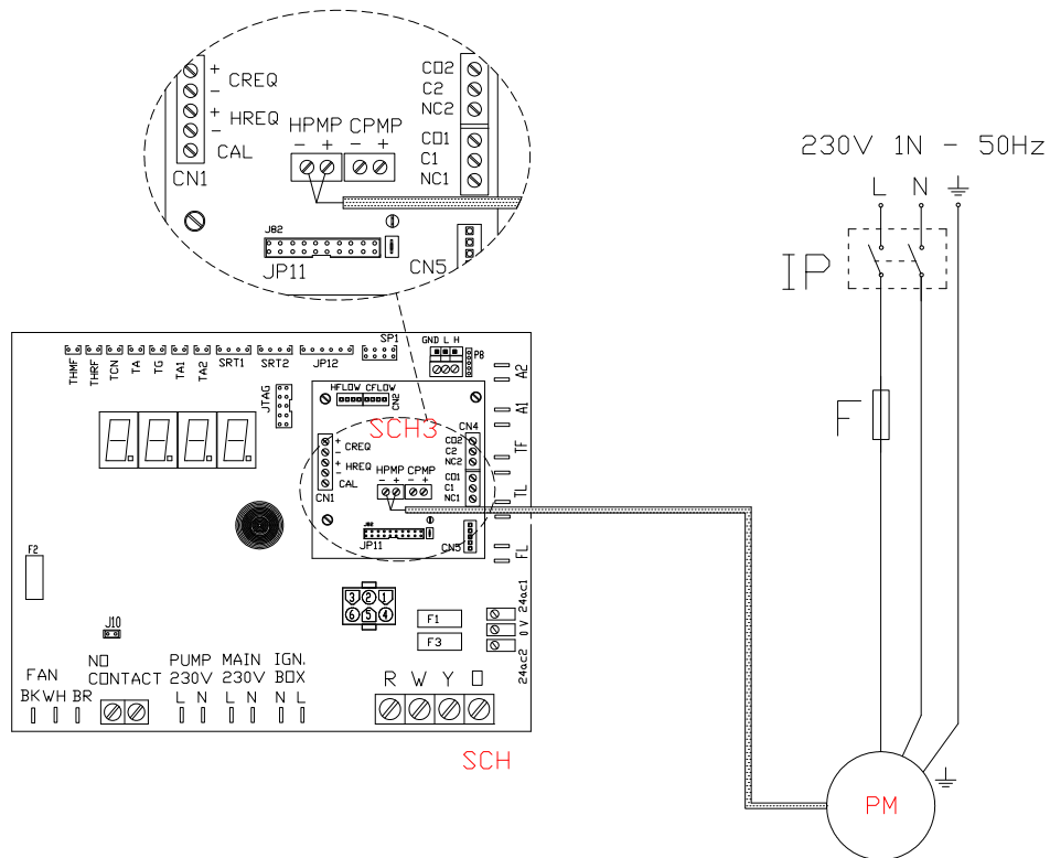
Figura 4.7 – Schema elettrico per il collegamento della pompa a portata variabile Wilo
