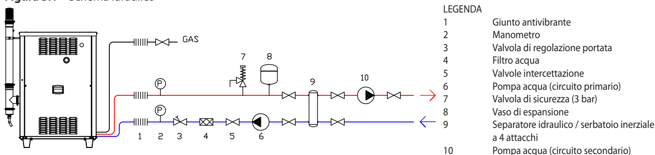
Figura 3.1 – Schema idraulico
