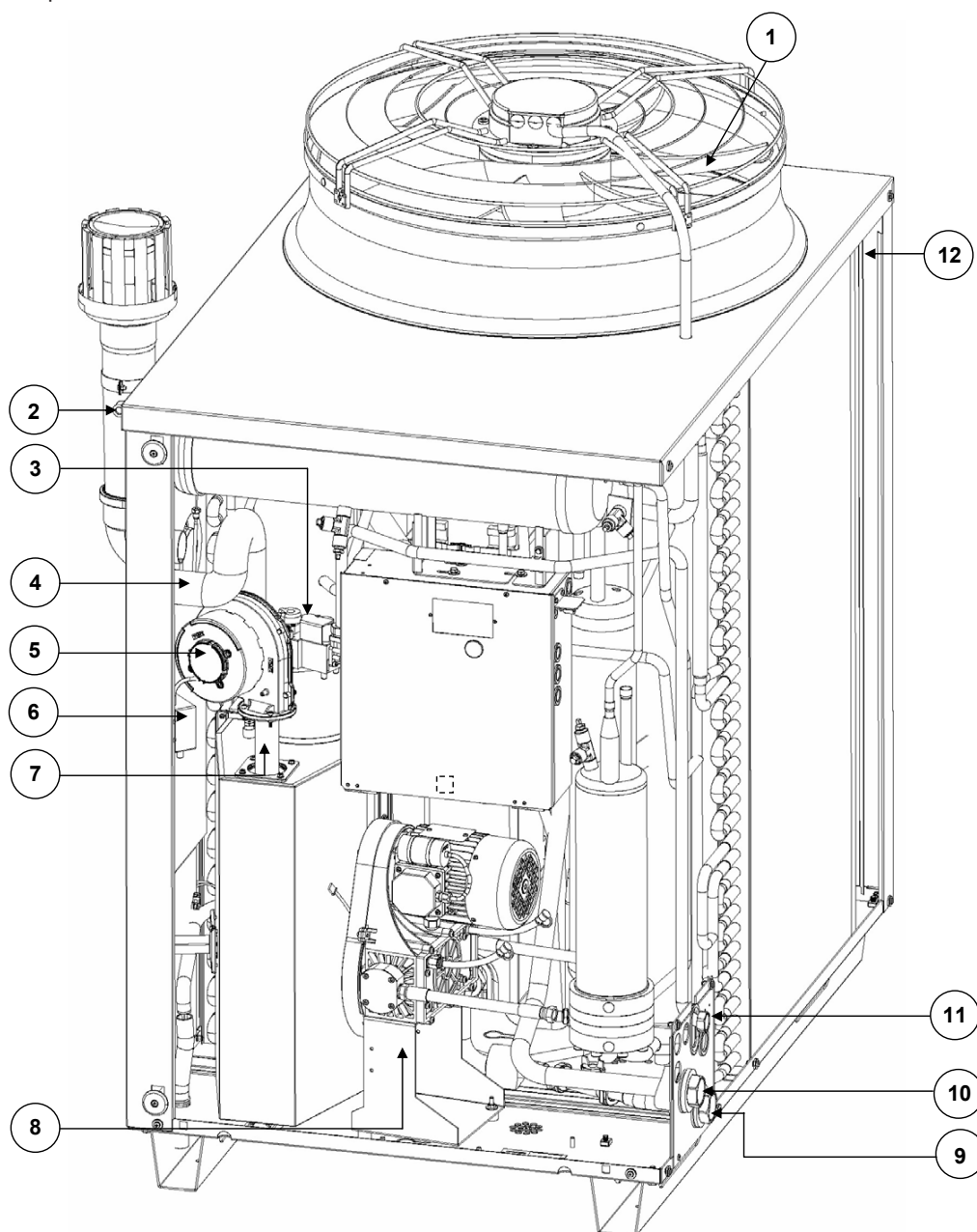
Figura 1.4 – Componenti interni vista frontale
