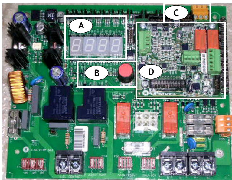
Figura 6.1 – Scheda elettronica a bordo unità GAHP
