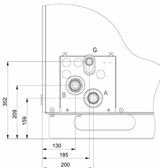
Figura 1.1 – Piastra servizi
