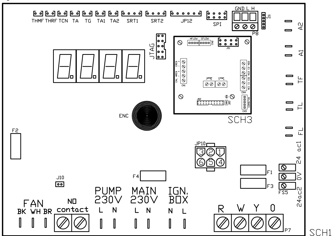
Figura 1.9 – Scheda elettronica S61
