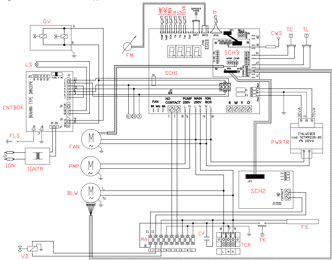
Figura 1.7 – Schema elettrico dell'apparecchio con ventilatore a basso consumo (S1)
