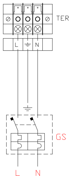
Figura 4.2 – Schema elettrico
