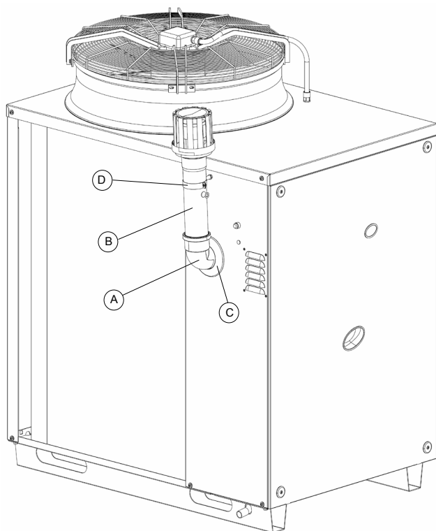
Figura 3.2 – Scarico fumi
