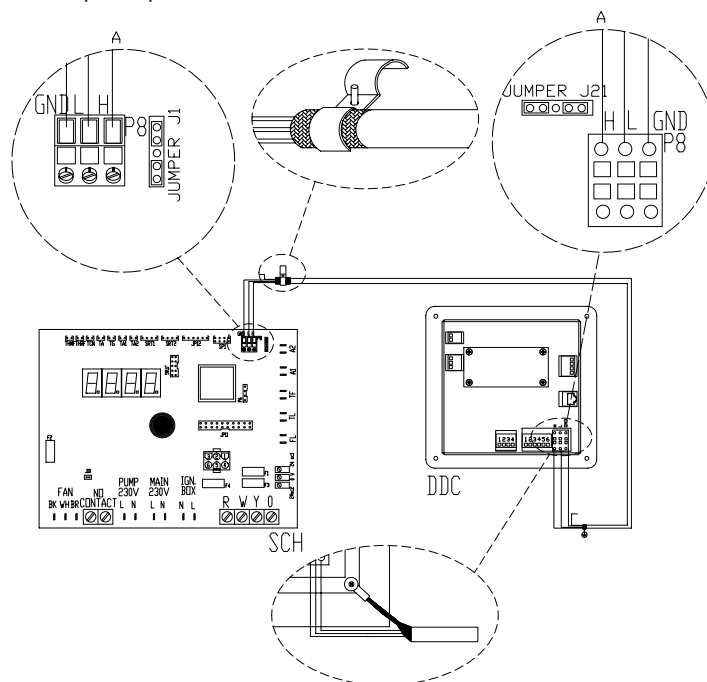
Figura 4.4 – Collegamento CAN-BUS per impianti con una unità
