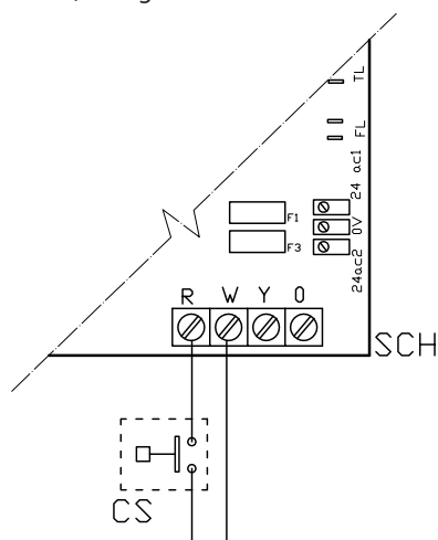
Figura 4.5 – Schema elettrico, collegamento consenso esterno
