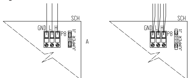
Figura 4.3 – Schema elettrico
