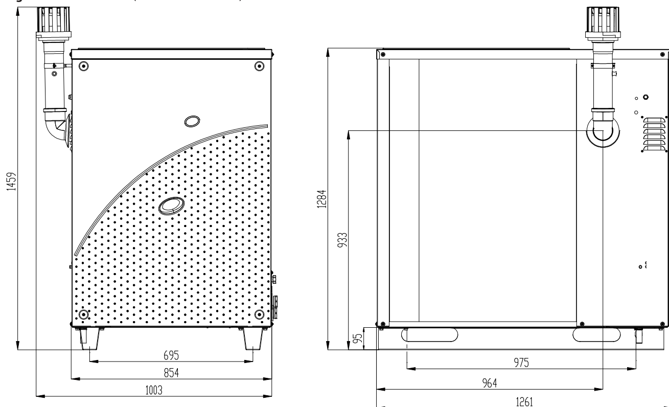
Figura 1.2 – Dimensioni (ventilatore standard)
