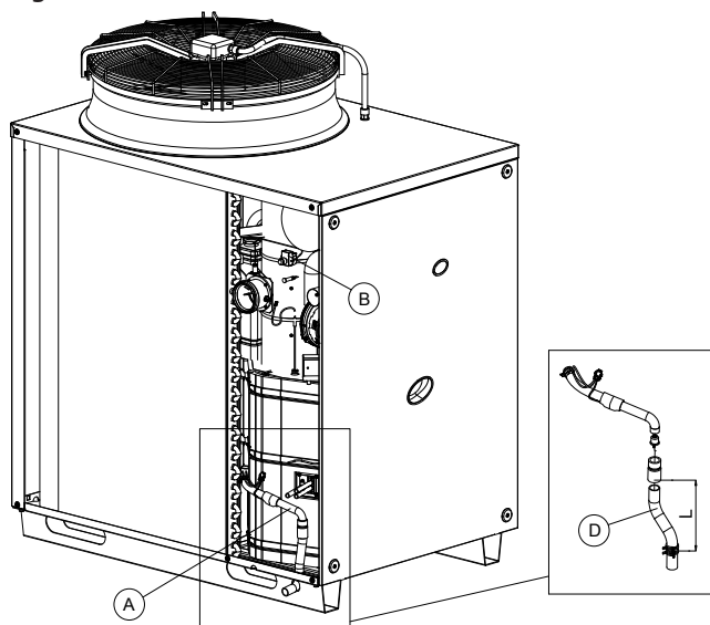
Figura 3.3 – Posizione scarico condensa
