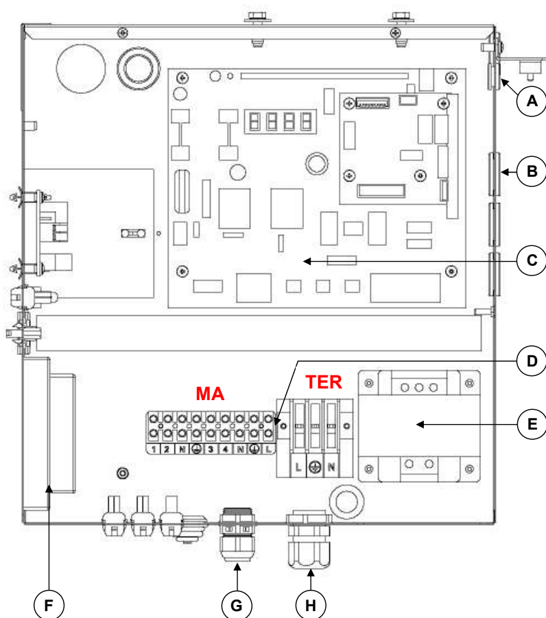
Figura 4.1 – Quadro Elettrico GAHP-A
