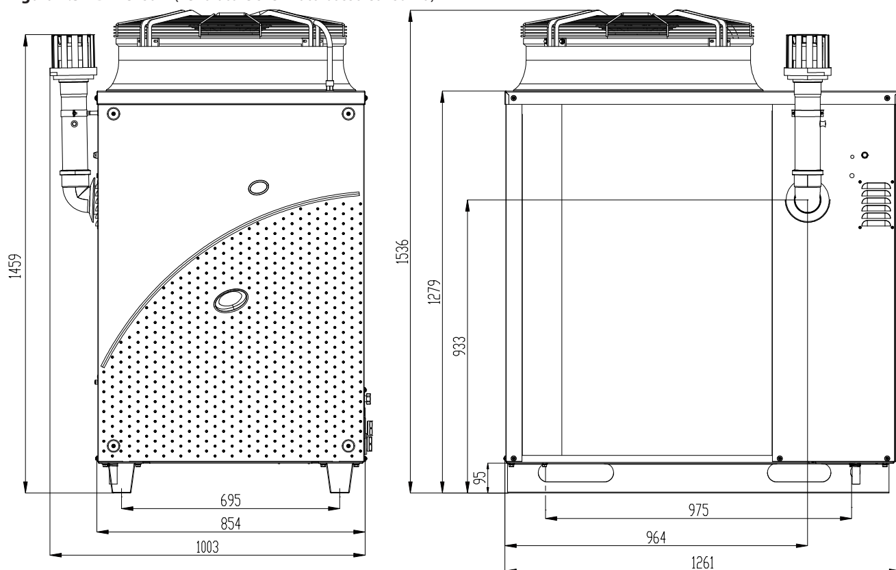
Figura 1.3 – Dimensioni (ventilatore silenzioso basso consumo)
