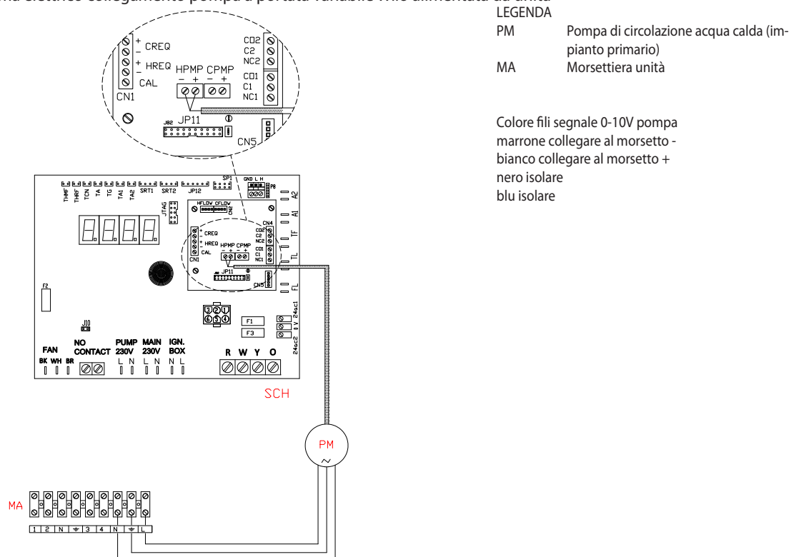
Figura 4.8 – Schema elettrico collegamento pompa a portata variabile Wilo alimentata da unità
