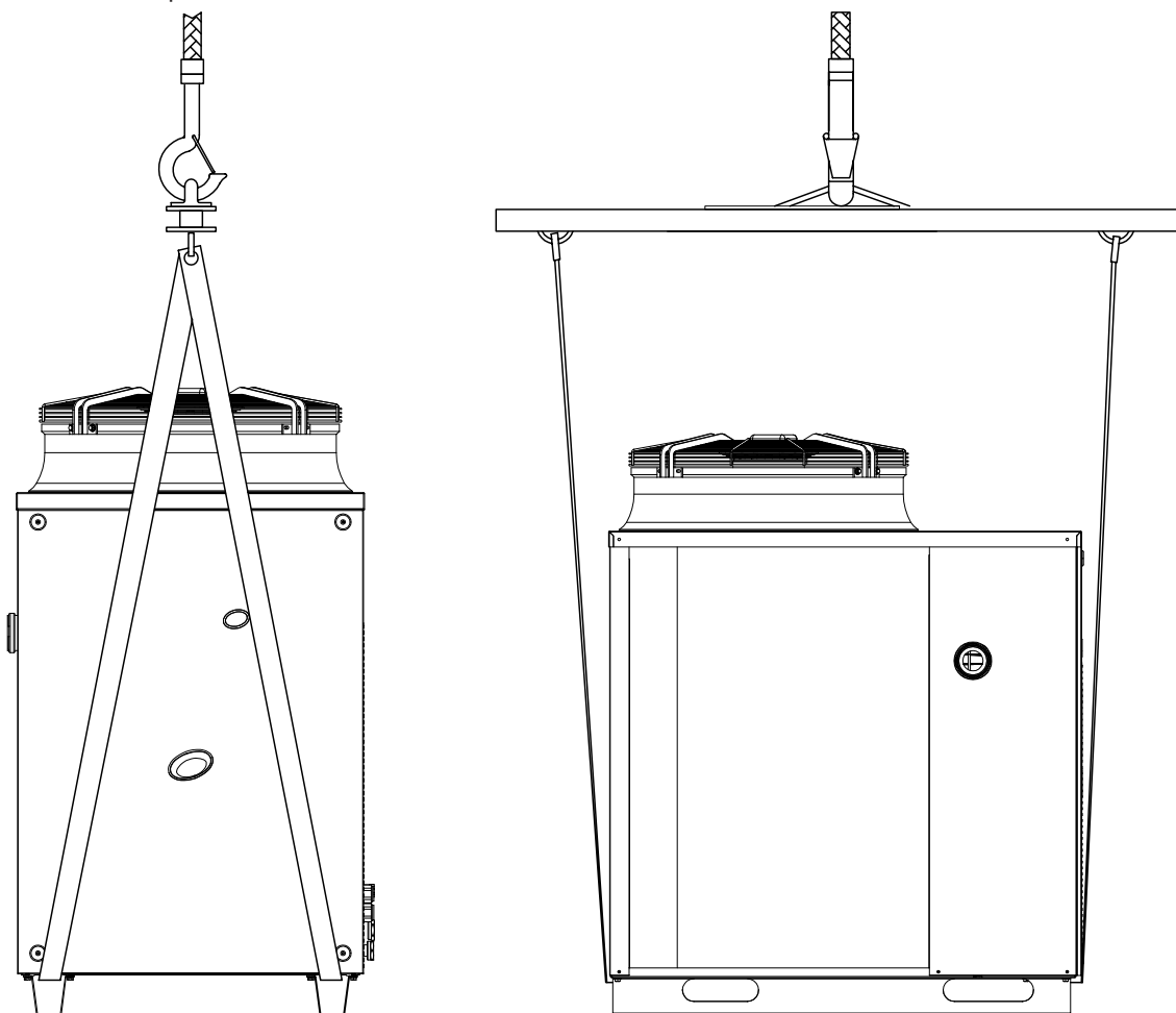
Figura 2.1 – Indicazioni per il sollevamento
