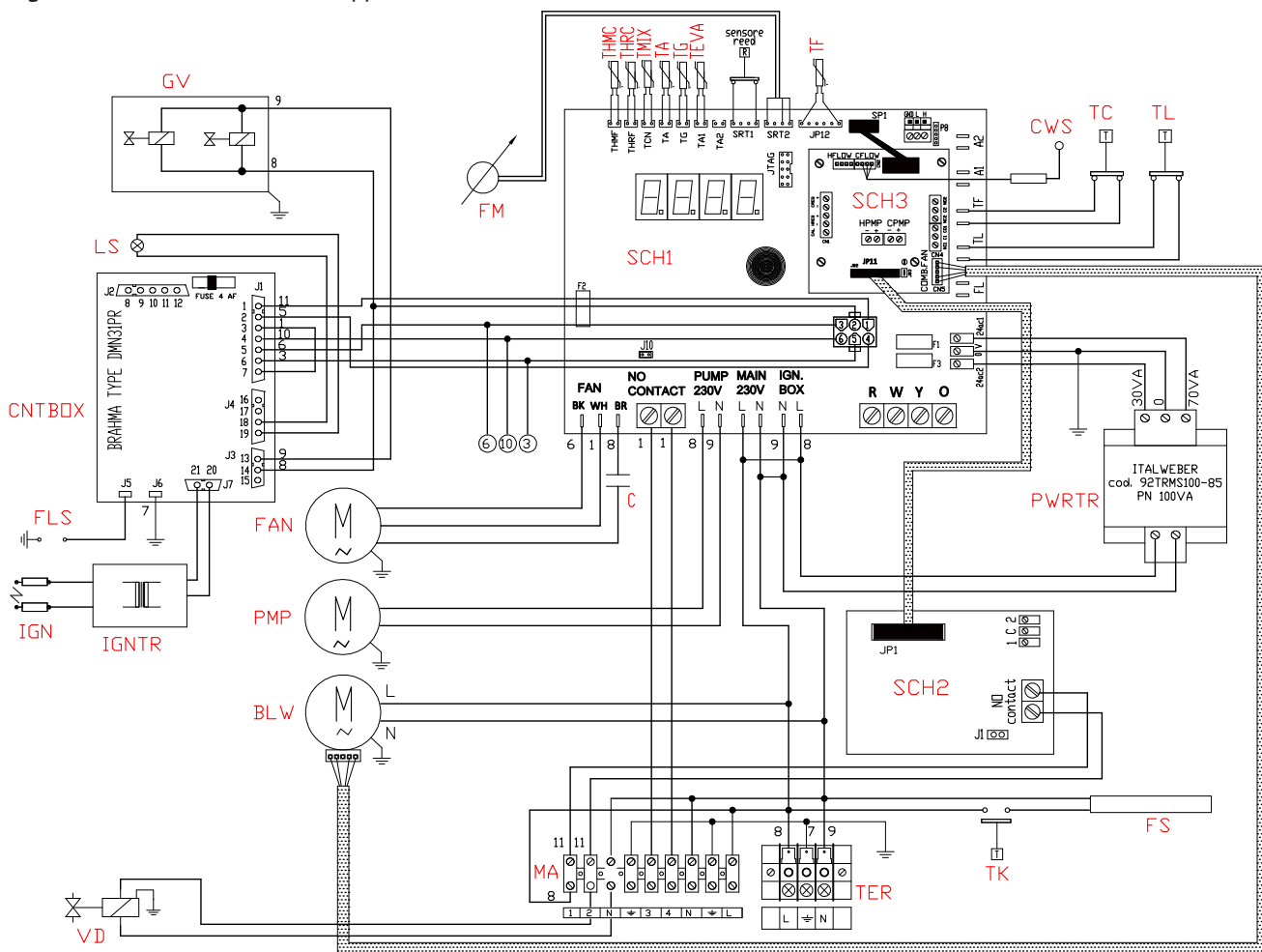
Figura 1.8 – Schema elettrico dell'apparecchio con ventilatore standard
