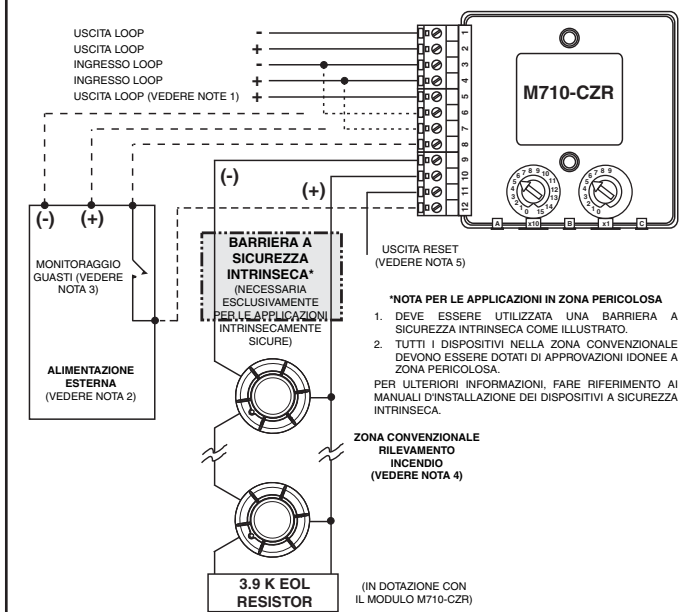
FIGURA 3: MODULO D'INTERFACCIA DI ZONA CONVENZIONALE M710-CZR
