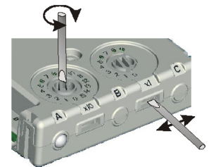
FIGURA 3: MÓDULO MONITOR PARA ZONAS CONVENCIONALES M710-CZR
