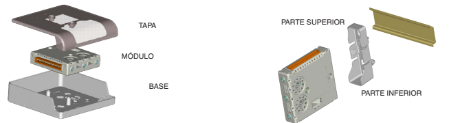
FIGURA 1: MÉTODOS DE MONTAJE DEL MÓDULO
