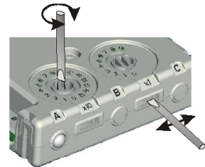
ABBILDUNG 3: M710-CZR ÜBERWACHUNGSMODUL FÜR GRENZWERTMELDER
