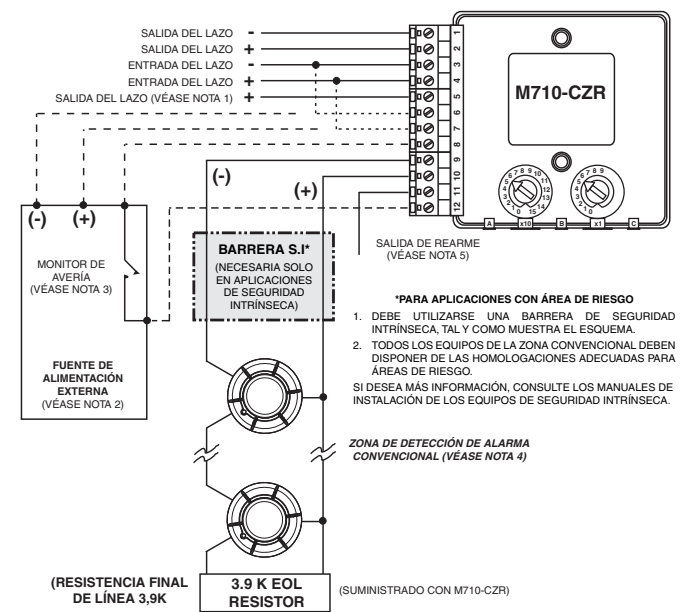
FIGURA 3: MÓDULO MONITOR PARA ZONAS CONVENCIONALES M710-CZR
