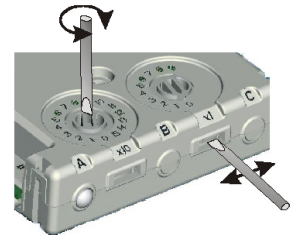
FIGURA 3: MODULO D'INTERFACCIA DI ZONA CONVENZIONALE M710-CZR
