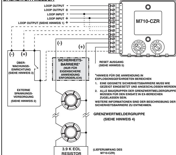
ABBILDUNG 3: M710-CZR ÜBERWACHUNGSMODUL FÜR GRENZWERTMELDER
