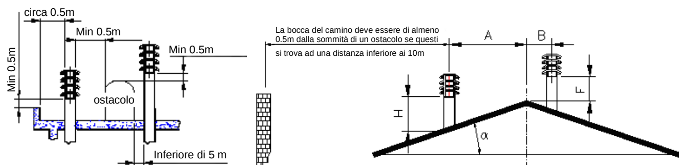
fig 3 Distanze e posizionamento comignoli
