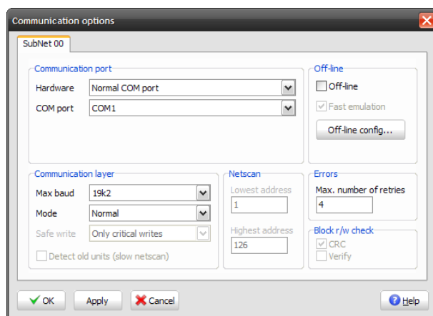
Figura 6.6: Opzioni di comunicazione di VariControl
