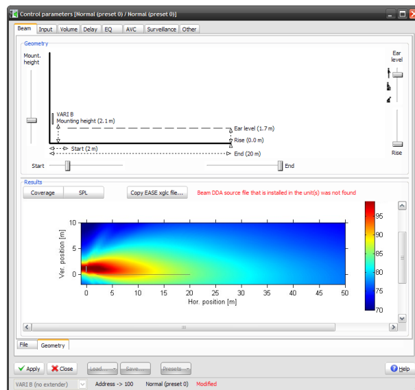
Figura 6.8: Riquadri Geometria e Risultati
