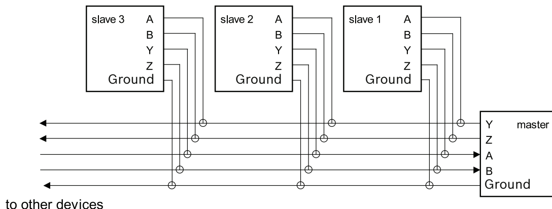
Figura 5.3: Struttura della rete RS-485
