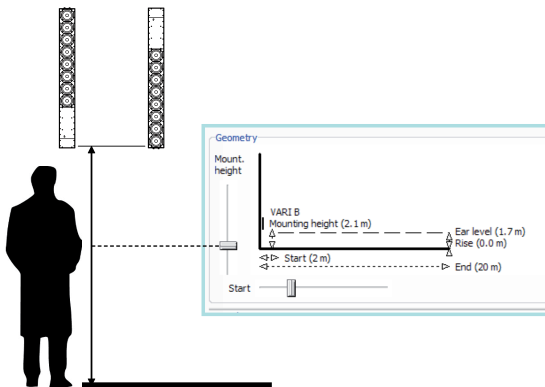
Figura 4.7: Altezza d'installazione
