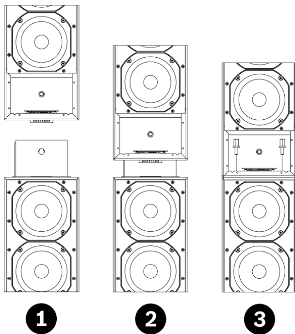
Figura 4.5: Allineamento dell'unità di estensione all'unità base
