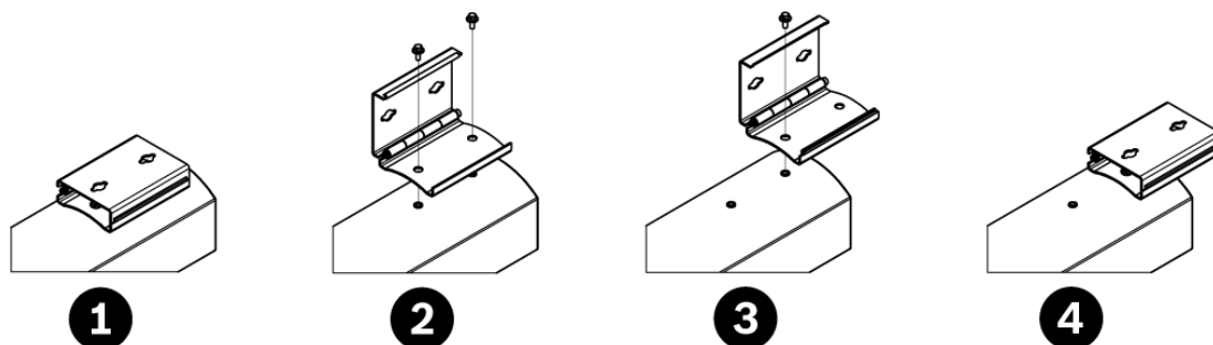
Figura 4.3: Riposizionamento della staffa
