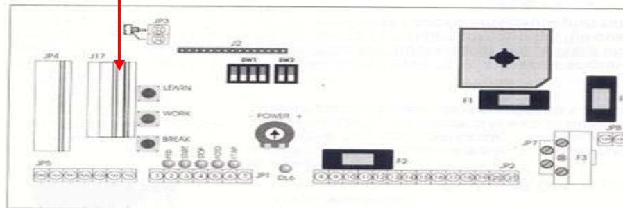
Connettore J17
