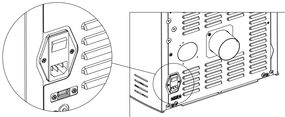
COLLEGAMENTO ELETTRICO DELLA STUFA
