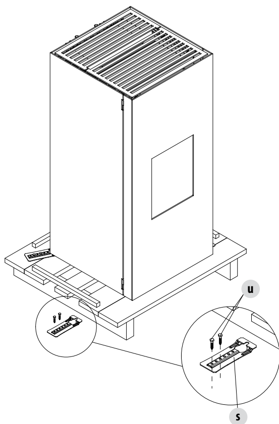
RIMOZIONE STAFFE DI FISSAGGIO
