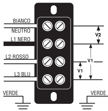
Modelli a 120/208 e 120/240 volt CA trifase, 50 Hz
