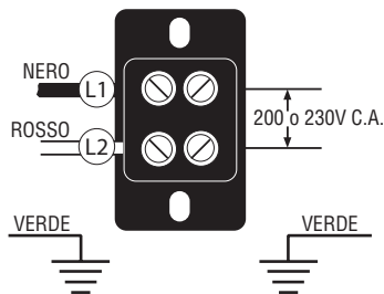
Modelli a 200 e 230 volt CA monofase, 60 Hz
