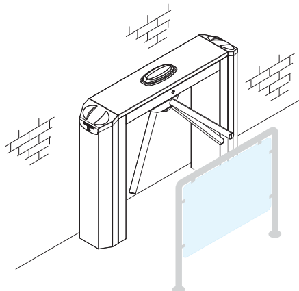
Installazione a ridosso muro
