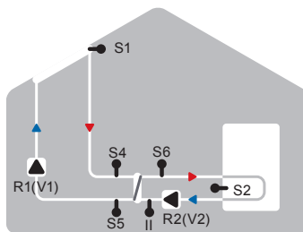
Solare con scambiatore
