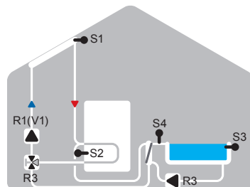
Solare piscina, accumulo, scambiatore
