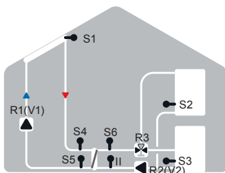
Solare con scambiatore e 2 accumulatori
