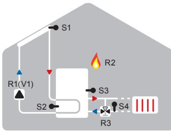
Solare con termostato e pre-riscaldamento
