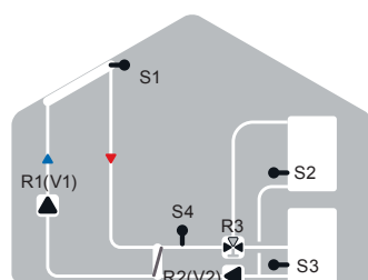
Solare con scambiatore 2 accumuli
