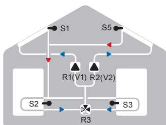
Solare est-ovest, 2 accumuli, 2 pompe
