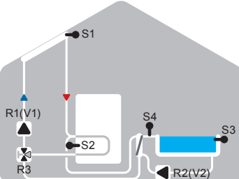
Solare con piscina, accumulo, scambiatore
