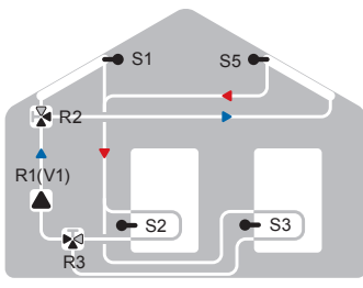
Solare est-ovest, 2 accumuli, 2 valvole
