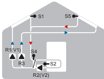
Solare est-ovest, scambiatore e 3 pompe
