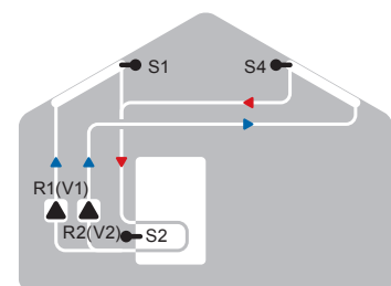
Solare + 2. collettori + Pompa
