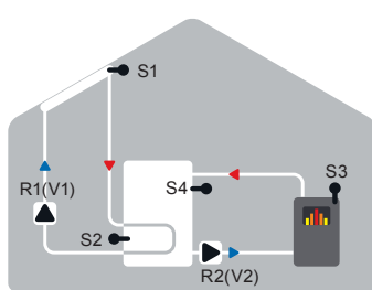
Solare accumulo e caldaia a legna
