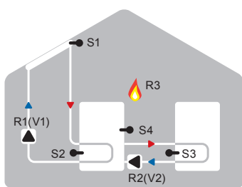
Solare con termostato e trasferimento
