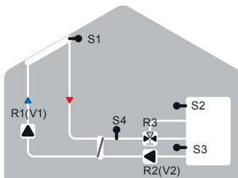
Solare con scambiatore 2 zone
