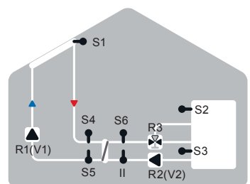
Solare con scambiatore e 2 zone
