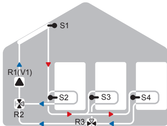
Solare 3 accumulatori e 3 valvole
