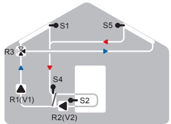
Solare est-ovest, scambiatore e 2 pompe
