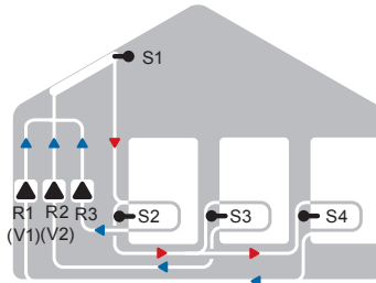
Solare con 3 accumuli e 3 pompe
