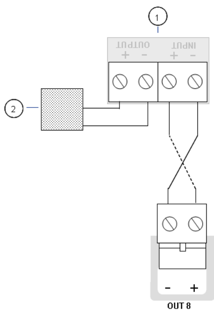
Figura 7: Connessione dell'attuatore di spegnimento della centrale
