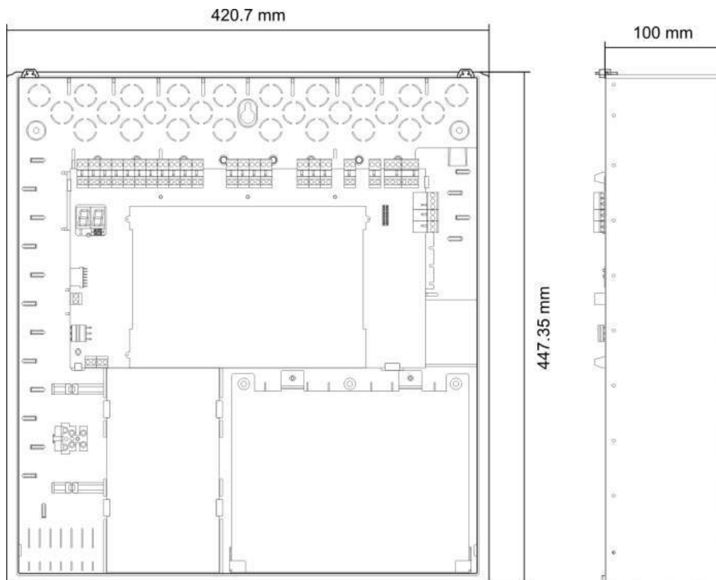
Figura 17: Armadietto della centrale senza coperchio
