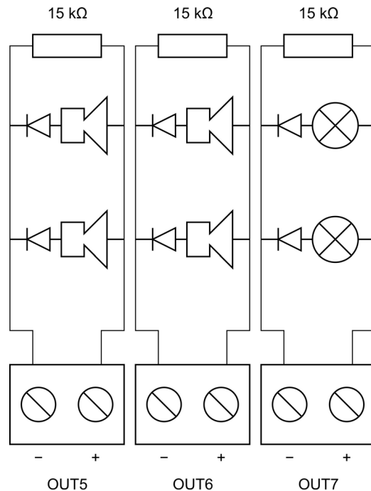
Figura 6: Uscite supervisionate standard della centrale
