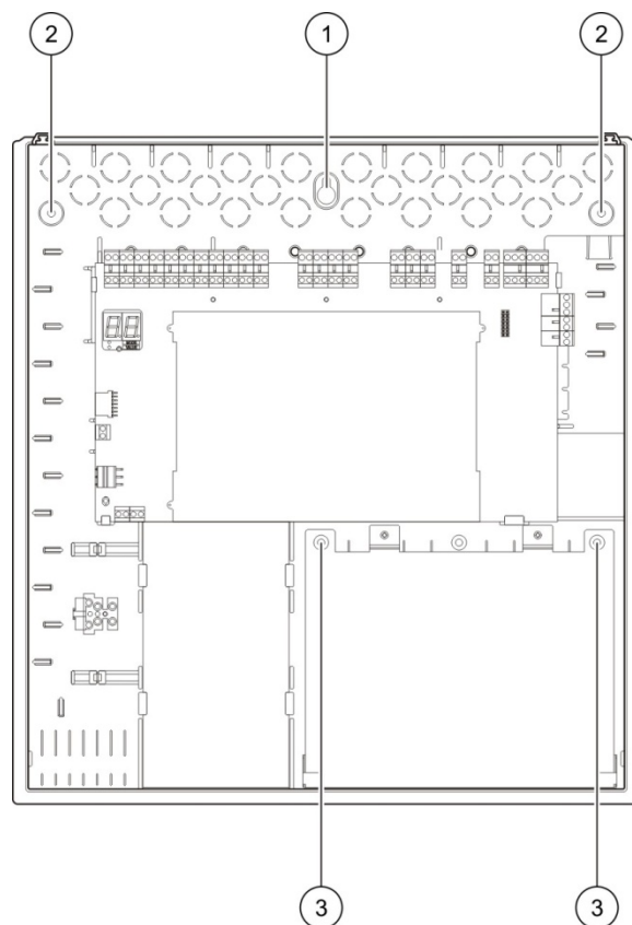
Figura 2: Posizioni dei fori di montaggio
