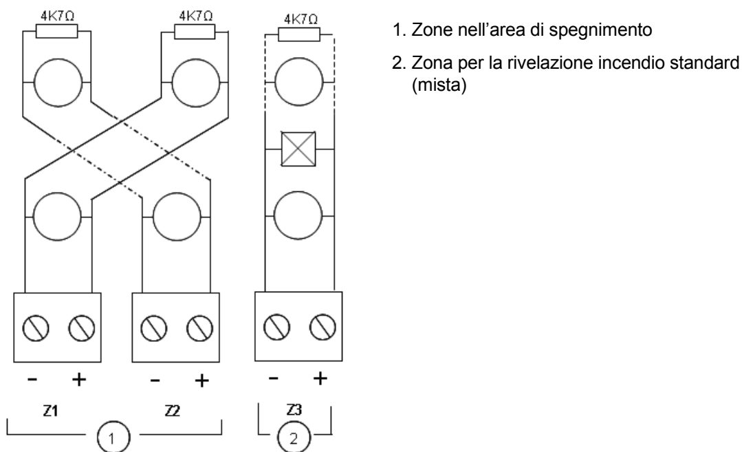
Figura 3: Collegamento delle zone per la configurazione predefinita
