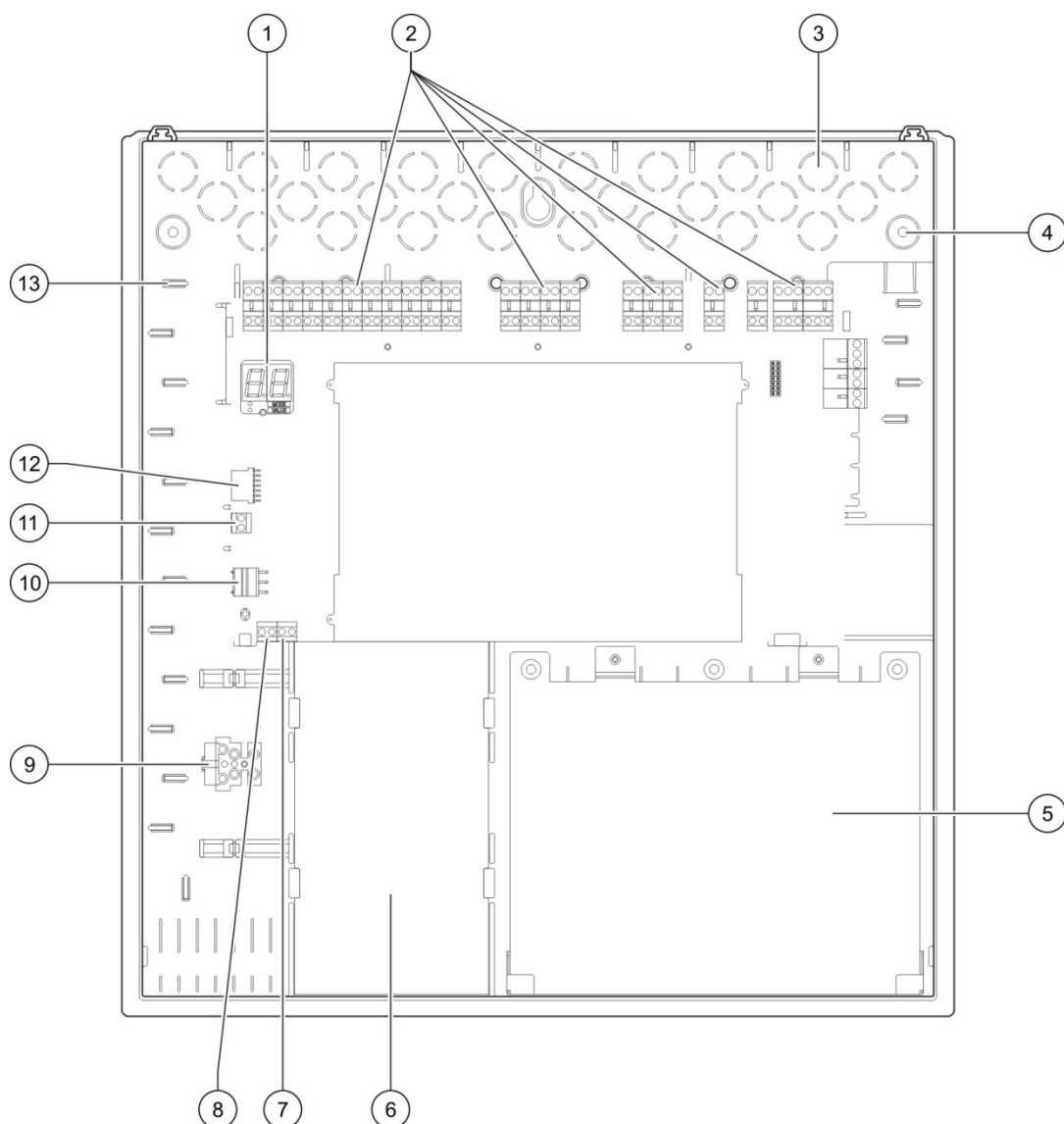
Figura 1: Layout dell'armadio della centrale
