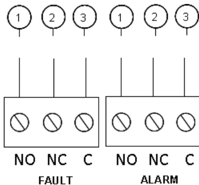
Figura 12: Collegamenti delle uscite relè di guasto e allarme
