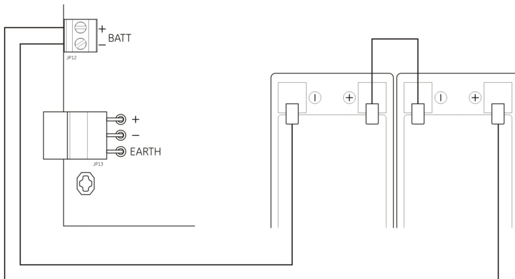
Figura 10: Collegamento delle batterie
