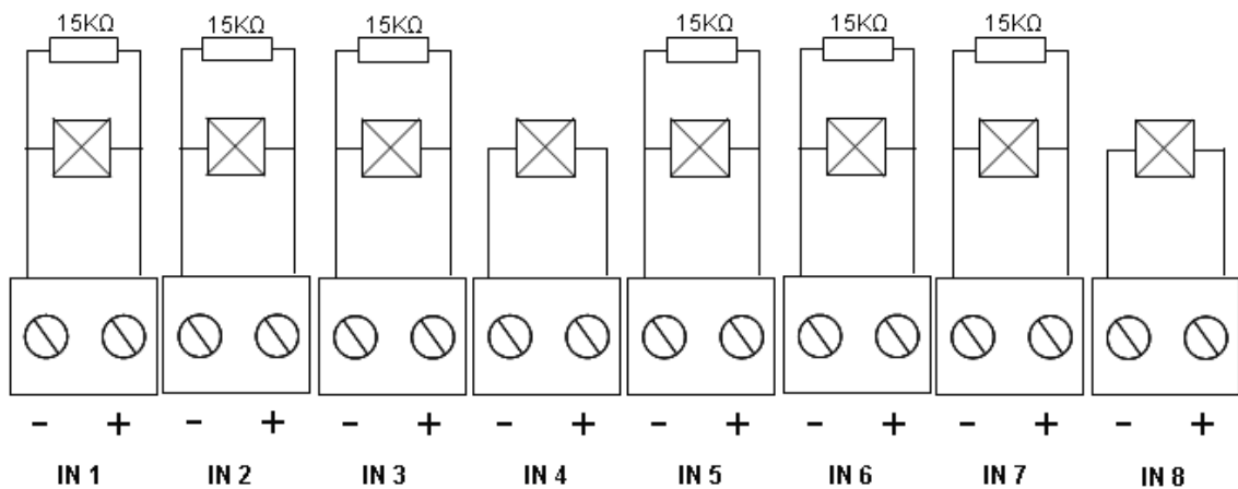
Figura 4: Collegamento degli ingressi
