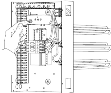
Figura 8 Reset della protezione termica
