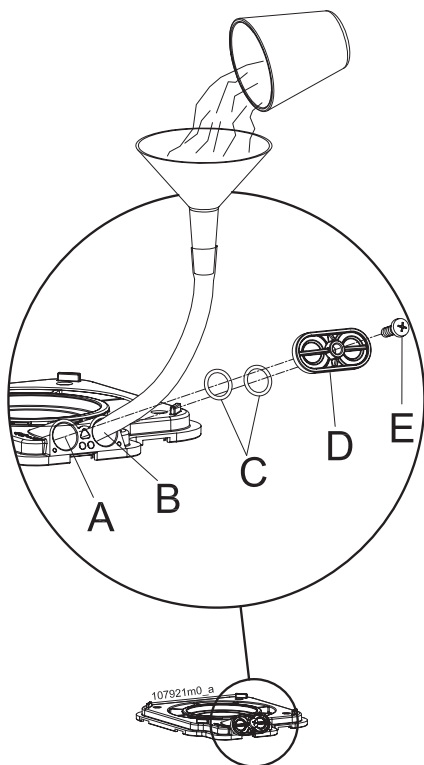
Figura 26 - Riempimento del sifone di scarico condensa
