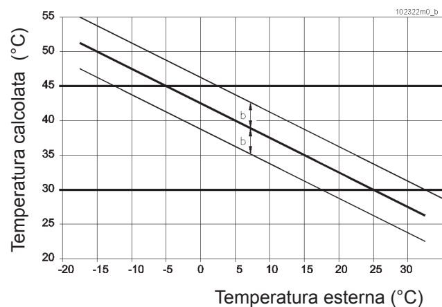
Figura 34 - Grafici della regolazione climatica per impianti a bassa temperatura
