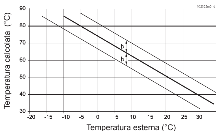
Figura 33 - Grafici della regolazione climatica per impianti ad alta temperatura
