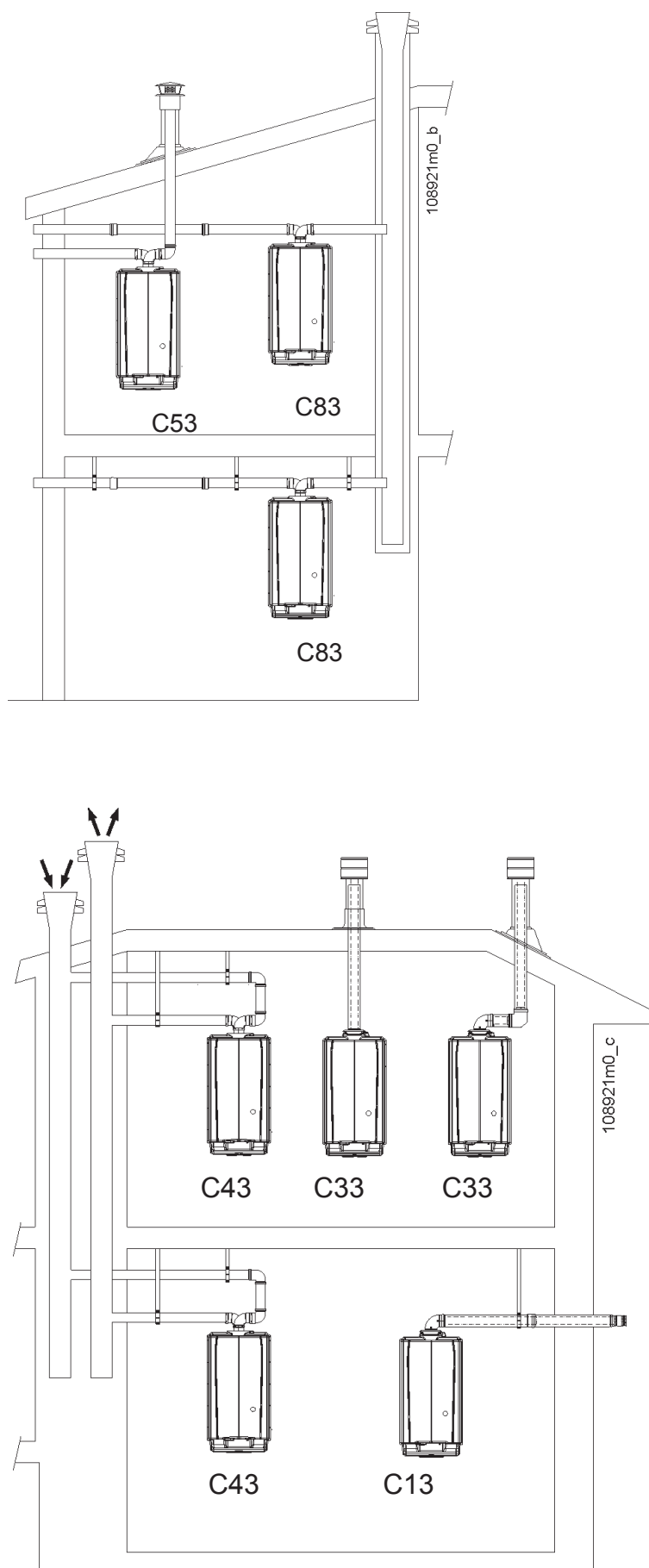
Figura 21 - Sistemi di scarico/aspirazione
