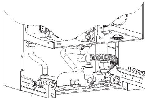
Figura 40 - Rubinetto di scarico circuito riscaldamento
