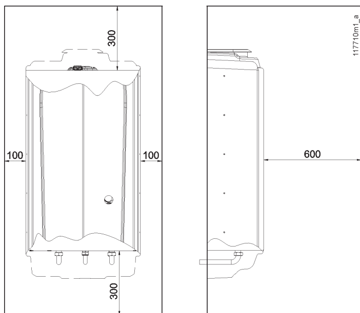
Figura 12 - Distanze minime di rispetto
