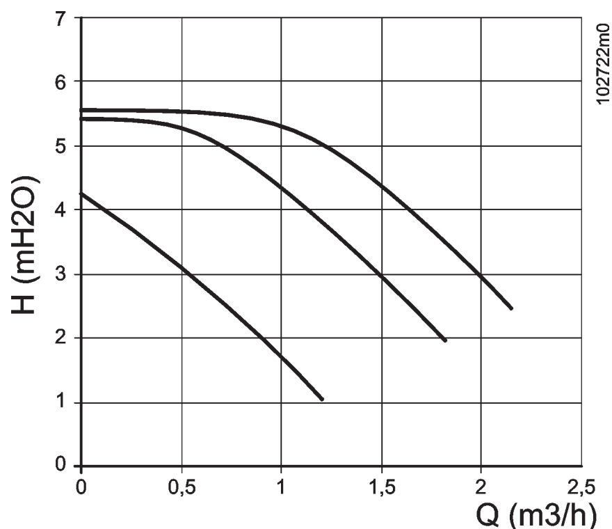
Figura 4 - Diagramma della prevalenza residua all'impianto per la caldaia CIELODENS 45C (con pompa integrata) (le tre curve corrispondono alle tre velocità del circolatore)
