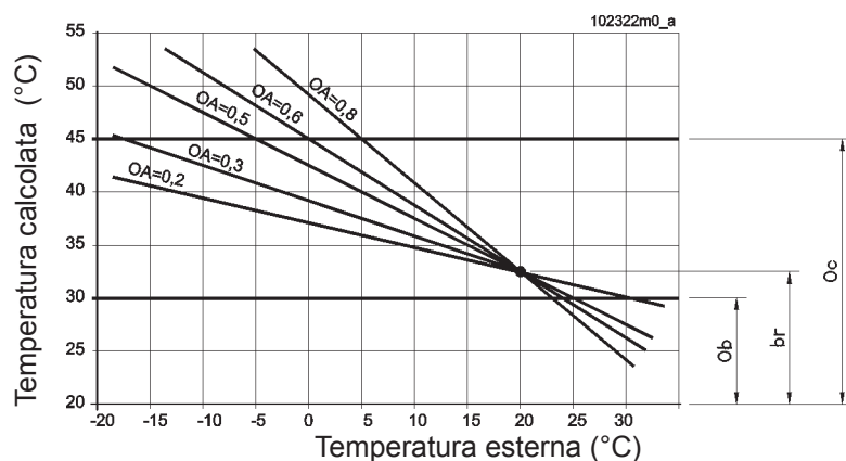
Figura 33 - Grafici della regolazione climatica per impianti ad alta temperatura
