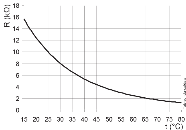
Figura 41- Curva sensori acqua
