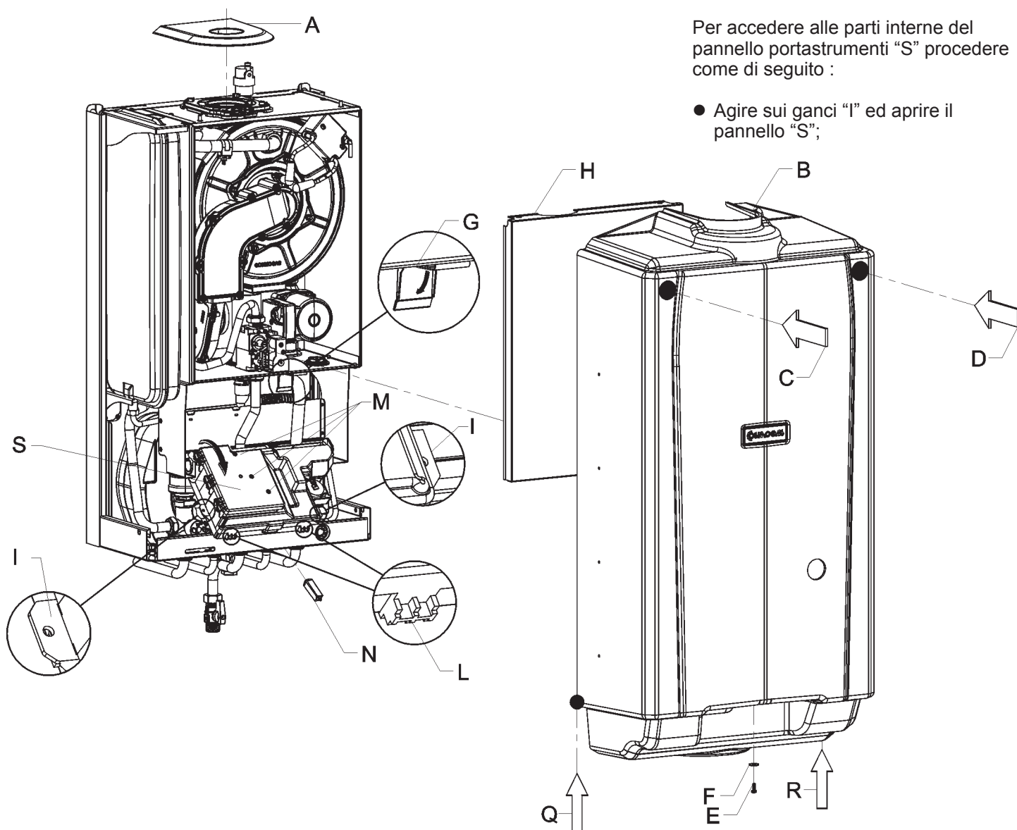
Figura 35 - Montaggio e smontaggio della mantellatura e accesso ai componenti interni
