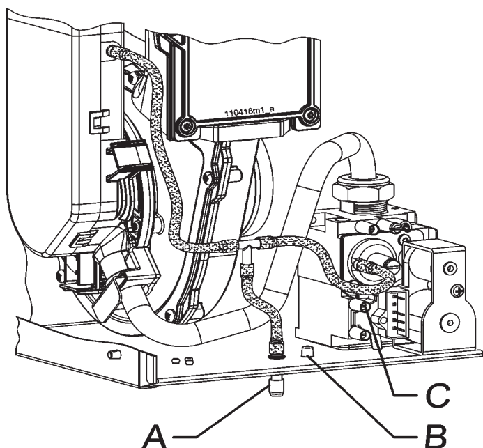
Figura 28 - Prese di pressione dell'aria comburente
