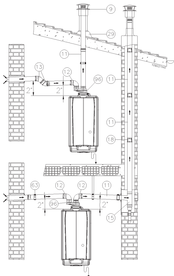
Figura 24 - Esempio di installazione “Sistema 80/80 PP”
