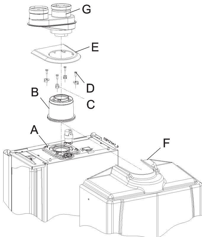
Figura 22 - Installazione del sistema “Sdoppiato 80/80 PP”
