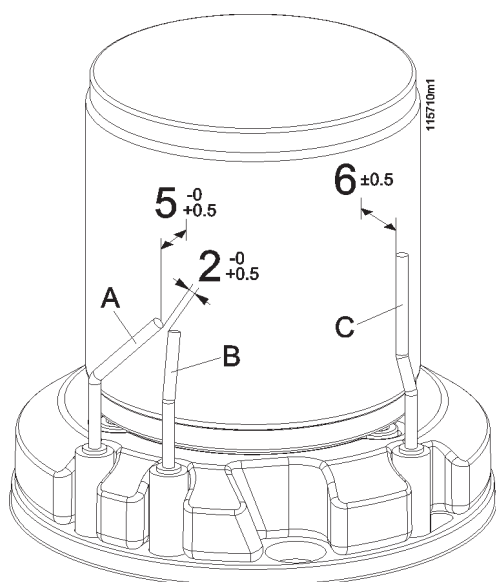
Figura 38 - posizionamento elettrodi sul bruciatore
