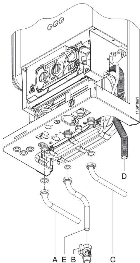
Figura 15 - Connessioni idrauliche e gas
