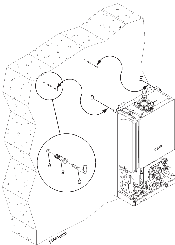
Figura 14 - Tasselli di sostegno
