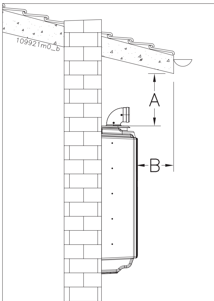
Figura 16 - Esempio di luogo parzialmente protetto
