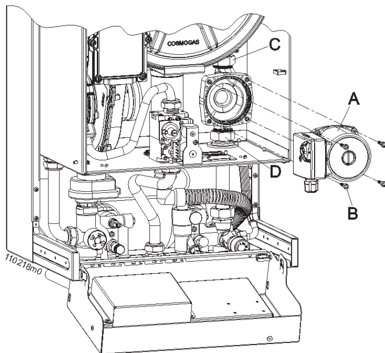
Figura 39 - Sostituzione del motore della pompa
