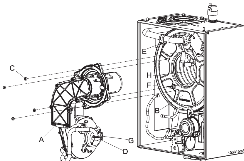
Figura 37 - Smontaggio gruppo ventilatore-bruciatore
