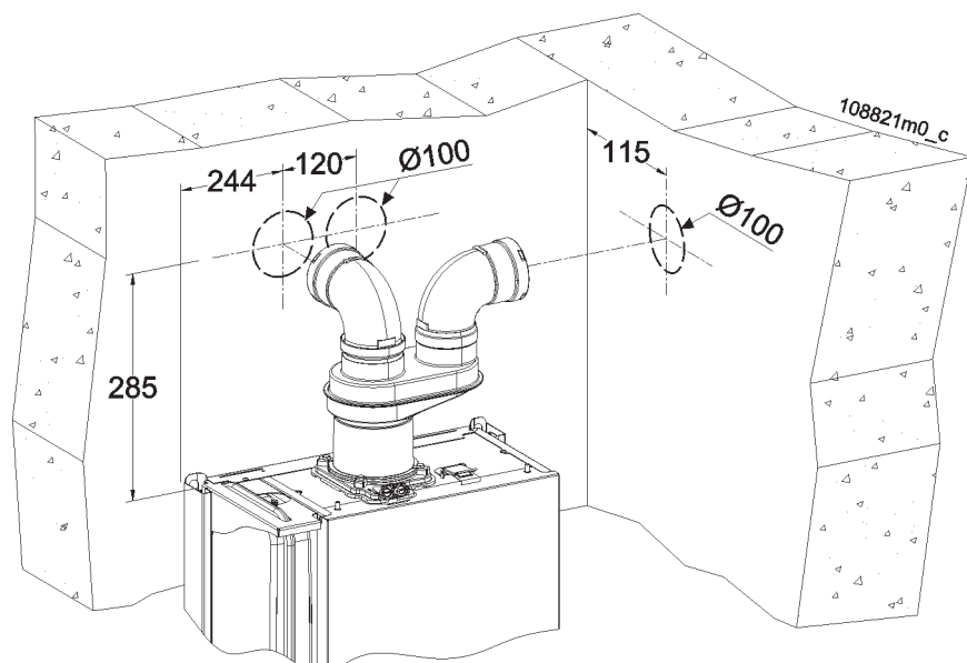
Figura 23 - Quote interassi dello scarico “Sdoppiato 80/80 PP”
