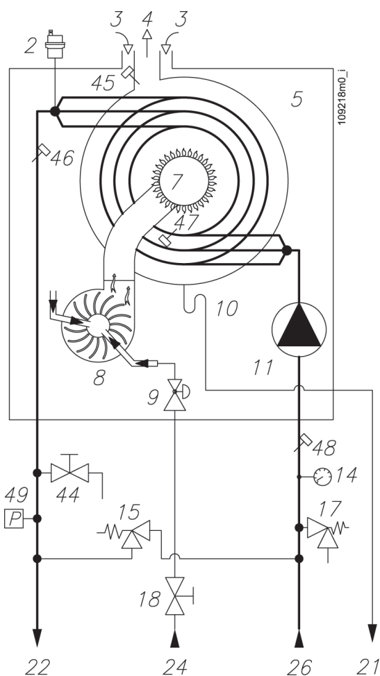
Figura 2 - Schema idraulico CIELODENS 45C
