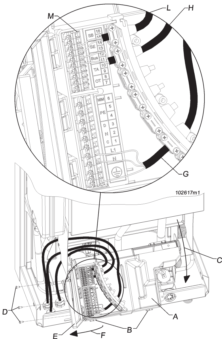
Figura 19 - Collegamenti elettrici
