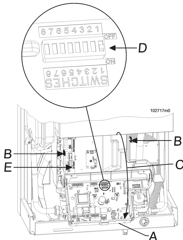
Figura 20 - Commutatori (SWITCHES) di adattamento caldaia
