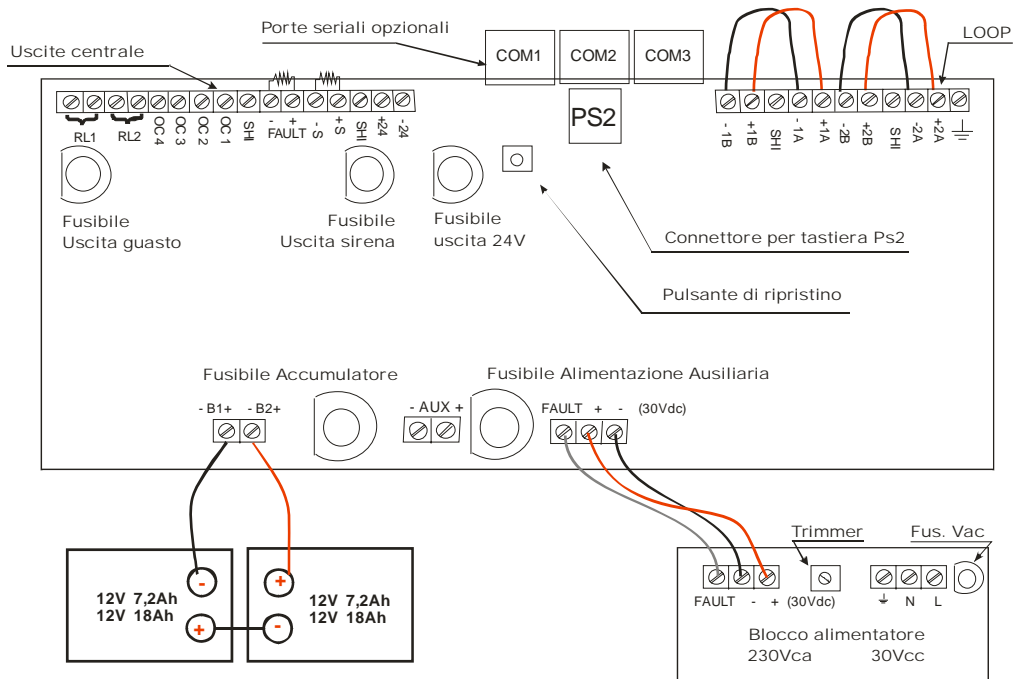
Fig. 2 – Descrizione della scheda elettronica della centrale.
