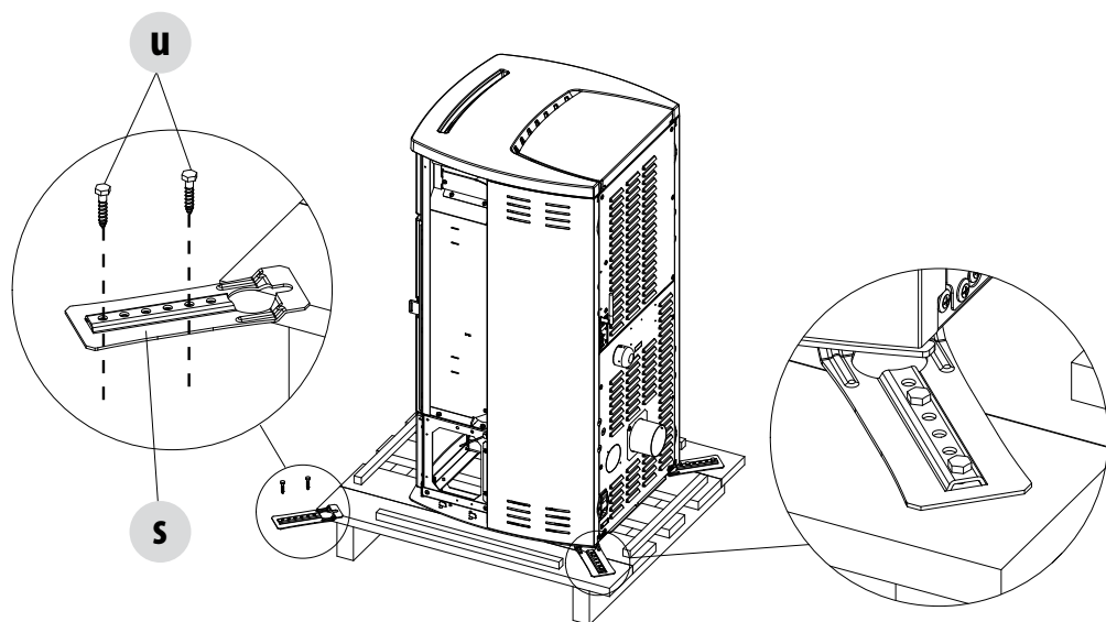
RIMOZIONE STAFFE DI FISSAGGIO (IN FIGURA STUFA EGO)
