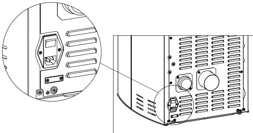
COLLEGAMENTO ELETTRICO DELLA STUFA
