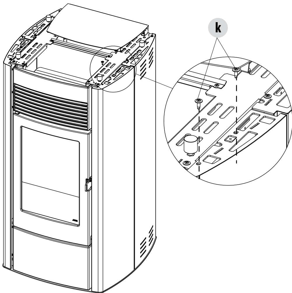
FISSAGGIO SUPERIORE DEL PANNELLO IN METALLO
