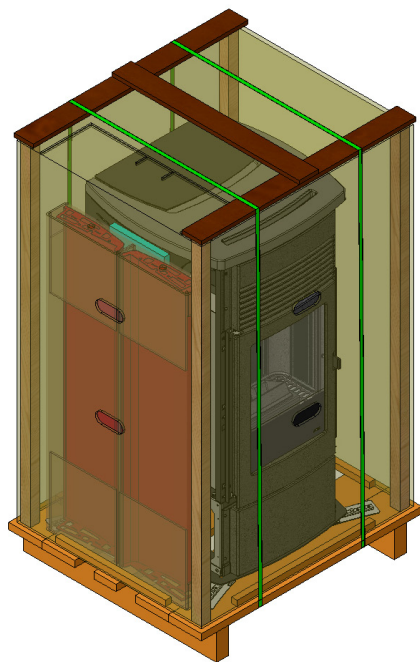
IMBALLO EGO CON RIVESTIMENTO IN ACCIAIO
