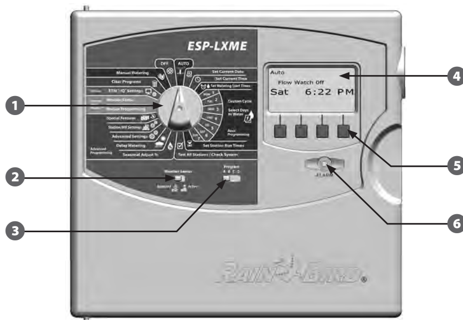
Figura A.1 - Funzioni del pannello frontale del programmatore ESP-LXME
