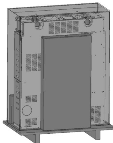
Figura 2 – Imballo stufa (vista posteriore)
