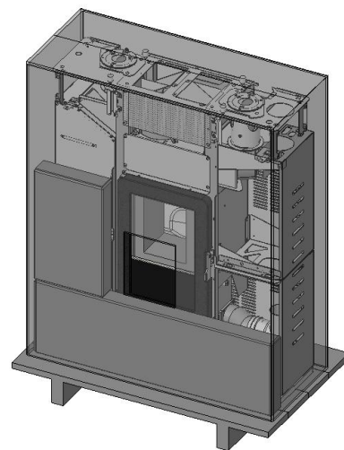
Figura 1 – Imballo stufa (vista frontale)
