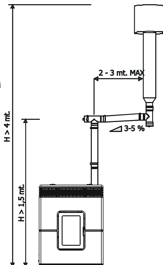
Esempio di installazione stufa a pellet
