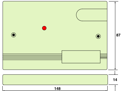
FIG. 3 FC410LI Placca Facia Plate Kurzschlussisolator Vorderseite
