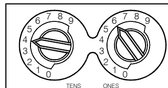
Figura 3. Selectores Giratorios de Dirección Decádicos
