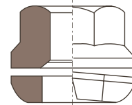
DIN 74361 B/C
