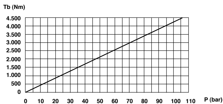
DIN 74361 H
