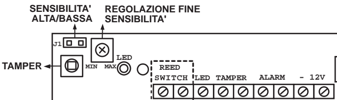
Figura 1: Schema Morsettiera
