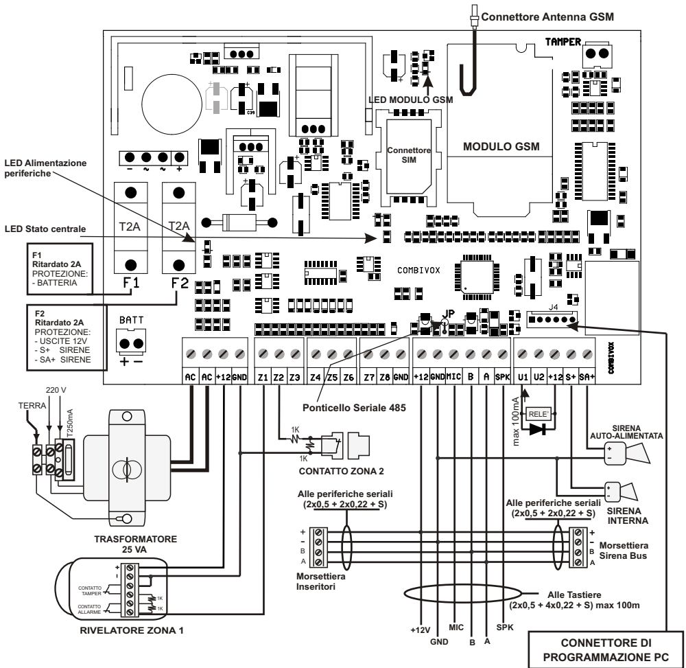
FIG. 8 SCHEMA DI CABLAGGIO ELISA
