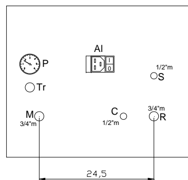
PANNELLO DI CONNESSIONE ALL'IMPIANTO CON GRUPPO STANDARD
