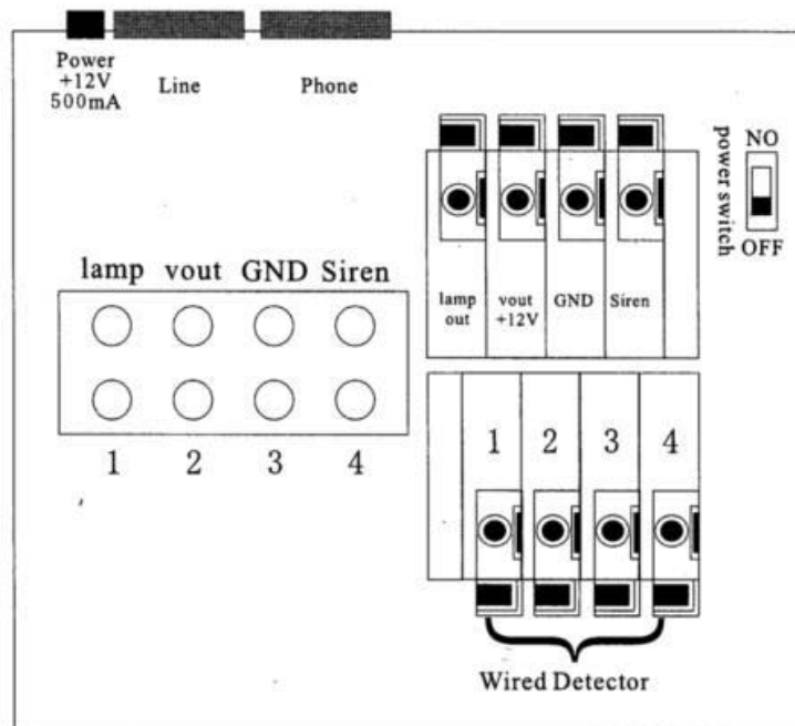
Fig. 3: Vista del retro del pannello
