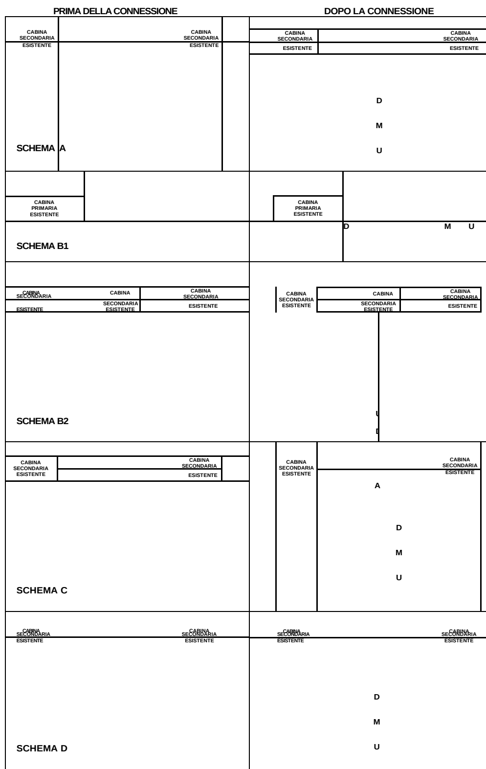
Figura 18 – Schemi di inserimento dell'impianto di Utente
