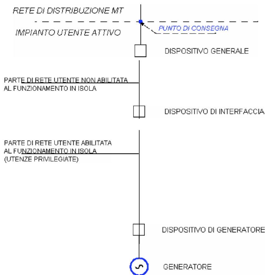
Figura 24 –Schema di principio della connessione di un impianto di produzione
