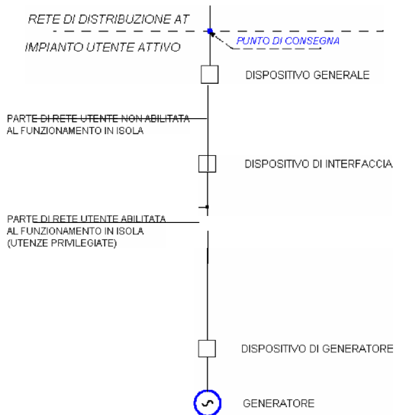
Figura 17 – Configurazione generale dell'impianto d'utenza attivo
