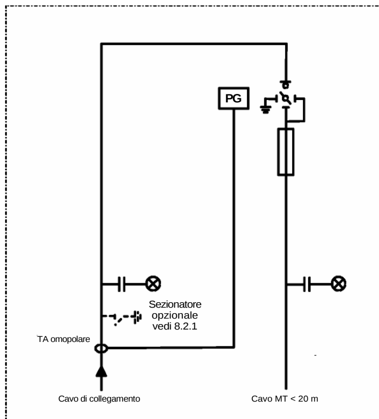
Figura 23 – DG semplificato per impianto passivo con un solo montante MT con a valle un solo trasformatore MT/BT di potenza nominale ≤ 400 kVA
