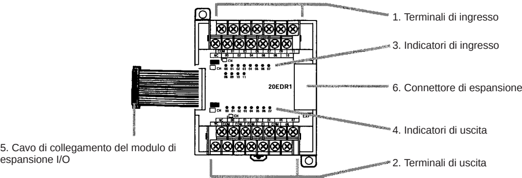
Modulo di espansione I/O con 20 terminali I/O
