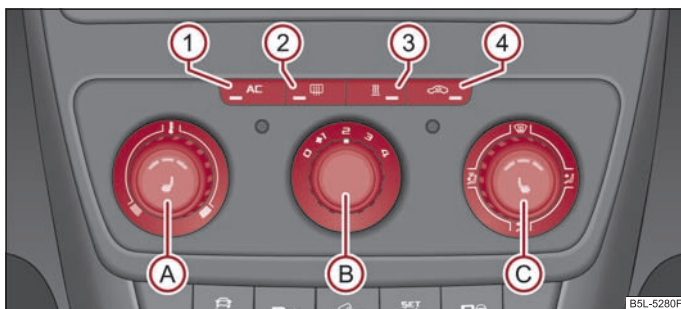
Fig. 5 Climatic: Elementi di comando
