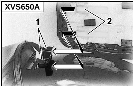
1. Supporto della sella (× 2)
